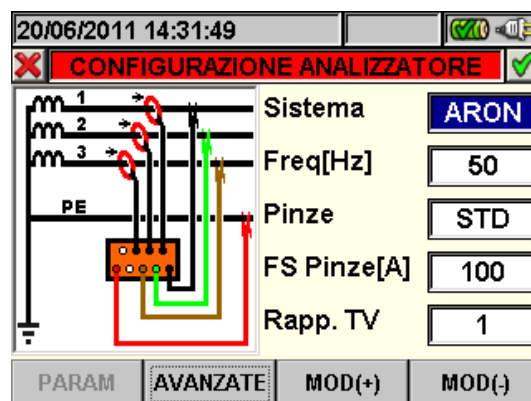
Fig. 82: Videata configurazione analizzatore per sistema Trifase ARON
