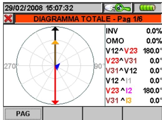
Fig. 149: Diagramma vettoriale totale in Sistema Trifase 3 fili o Sistema Aron
