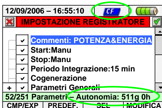
Fig. 179: Esempio di uso della memoria esterna - presenza Compact Flash
