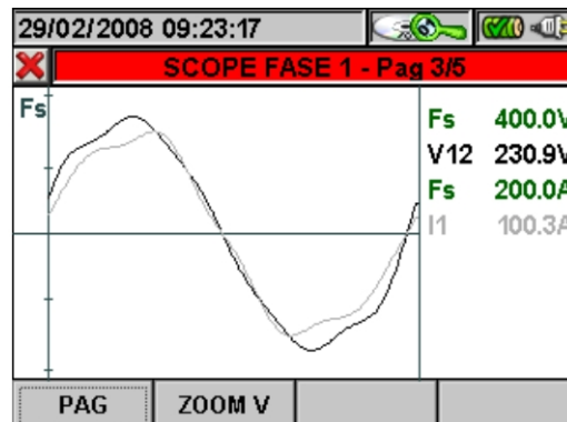
Fig. 132: Scope Fase 1 in Sistema Trifase 3 fili o Sistema Aron
