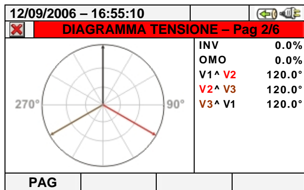
Fig. 70: Diagramma vettoriale tensioni per sistemi 4-fili
