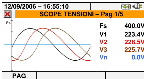
Fig. 42: Videata forme d'onda delle tensioni per sistema trifase 4-fili
