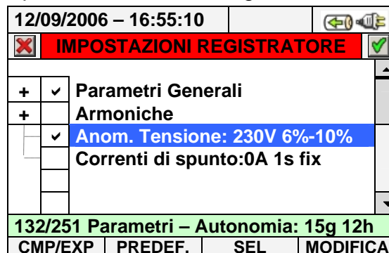
Fig. 99: Videata Anomalie di Tensione
