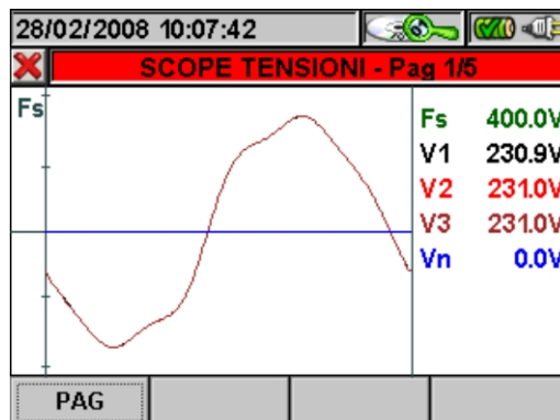
Fig. 126: Scope Tensioni in Sistema Trifase 4 fili
