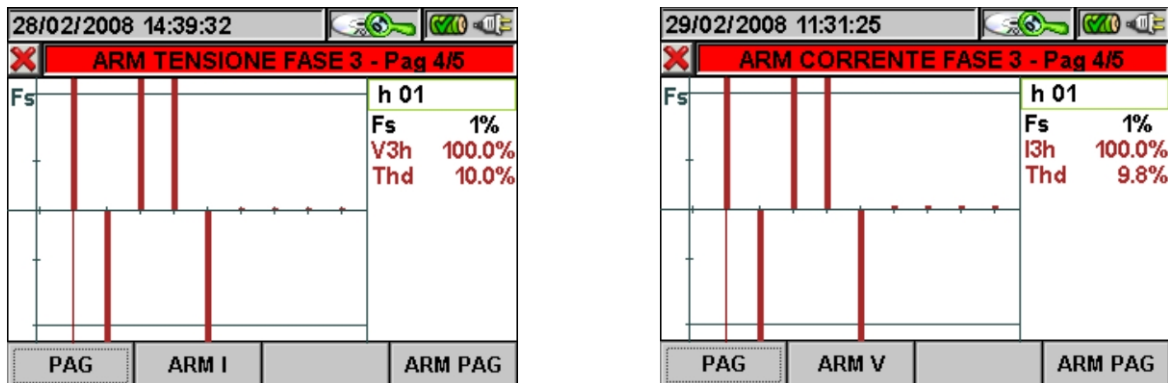
Fig. 144: Armoniche Fase3 in Sistema Trifase 4 fili
