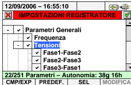
Fig. 94: Sottolivello Parametri Generali - Caso Trifase ARON
