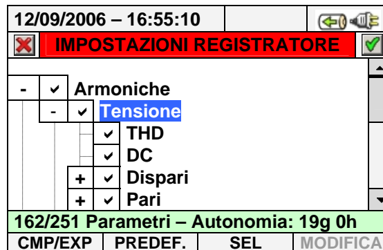
Fig. 95: Sottolivello Armoniche – selezione iniziale parametri
