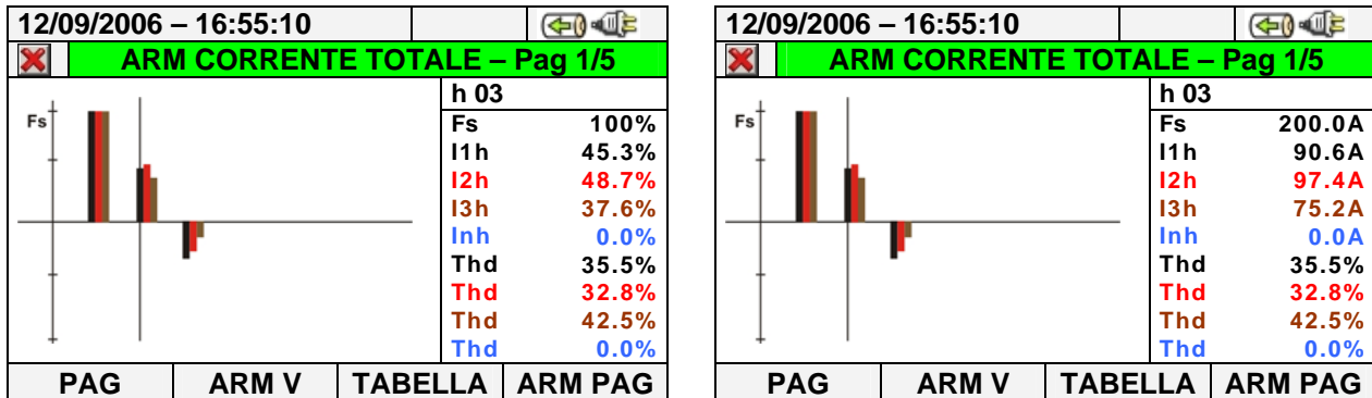
Fig. 56: Analisi armonica correnti in valore percentuale/assoluto sistemi 4-fili
