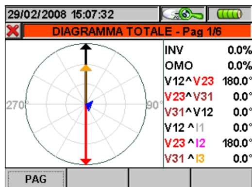
Fig. 150: Diagramma vettoriale di fase in Sistema Monofase
