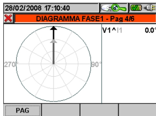
Fig. 156: Diagramma vettoriale Fase2 in Sistema Trifase 4 fili
