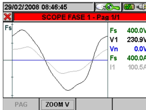
Fig. 128: Scope Tensione e Corrente in Sistema Monofase
