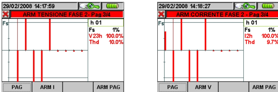
Fig. 143: Armoniche Fase2 in Sistema Trifase 3 fili o Sistema Aron
