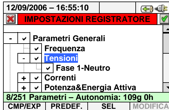
Fig. 91: Sottolivello Parametri Generali - Caso Monofase
