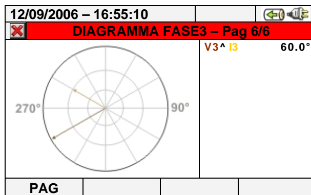
Fig. 75: Diagramma vettoriale tensione-corrente fase L3 per sistemi 4-fili
