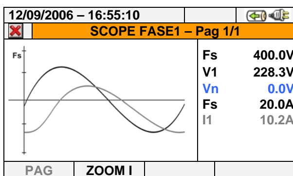
Fig. 44: Videata forme d'onda tensione/corrente per sistema Monofase
