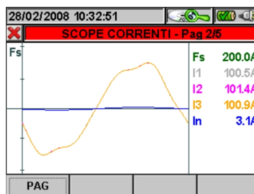
Fig. 129: Scope Correnti in Sistema Trifase 4 fili
