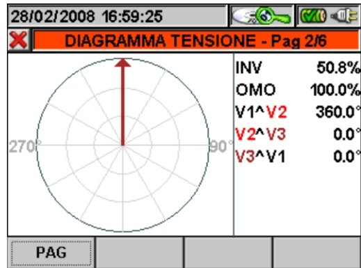
Fig. 151: Diagramma vettoriale Tensione in Sistema Trifase 4 fili
