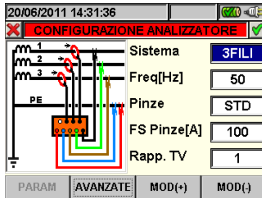
Fig. 81: Videata configurazione analizzatore per sistema Trifase 3-fili
