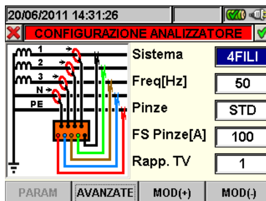
Fig. 80: Videata configurazione analizzatore per sistema Trifase 4-fili
