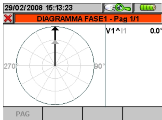
Fig. 152: Diagramma vettoriale Tensione in Sistema Trifase 3 fili o Sistema Aron
