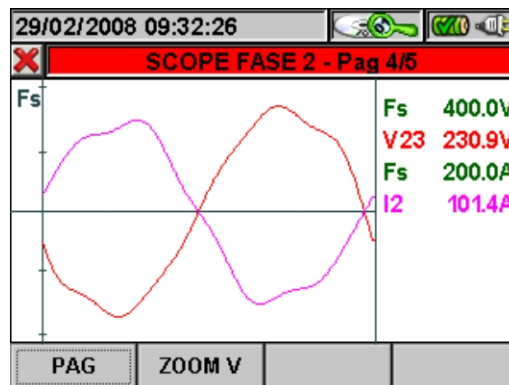
Fig. 134: Scope Fase 2 in Sistema Trifase 3 fili o Sistema Aron
