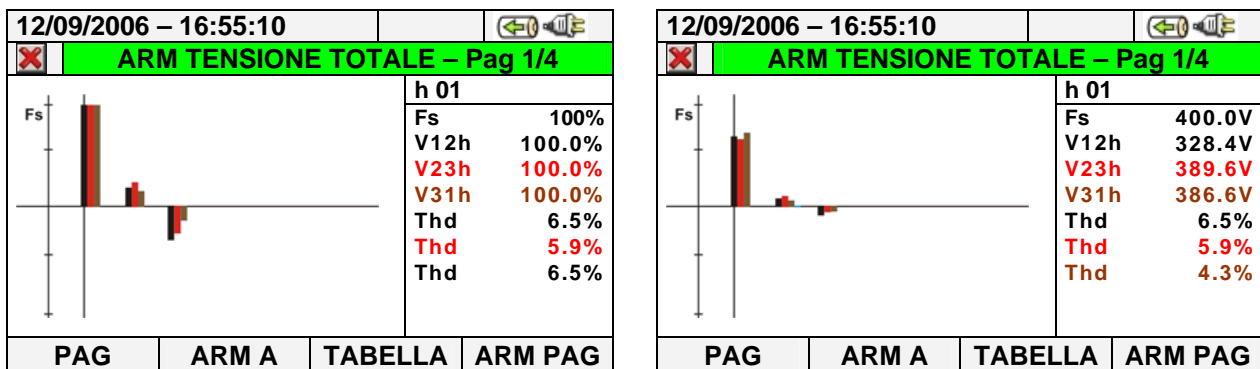
Fig. 54: Analisi armonica tensioni in valore percentuale/assoluto per sistemi 3-fili e ARON
