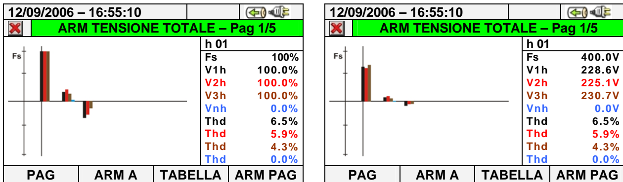
Fig. 53: Analisi armonica tensioni in valore percentuale/assoluto per sistemi trifase 4-fili
