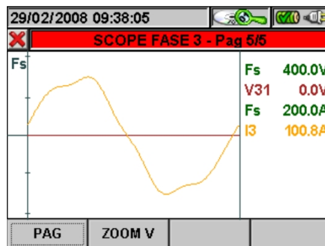
Fig. 136: Scope Fase 3 in Sistema Trifase 3 fili o Sistema Aron
