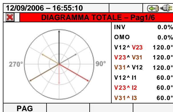
Fig. 68: Diagramma vettoriale totale per sistemi 3-fili e ARON
