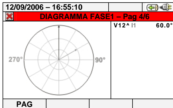
Fig. 76: Diagramma vettoriale tensione-corrente fase L1 per sistemi 3-fili e ARON
