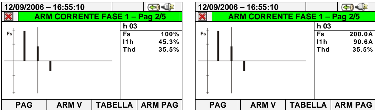
Fig. 66: Analisi armonica Corrente I1 in valore percentuale e assoluto per sistema 4-fili
