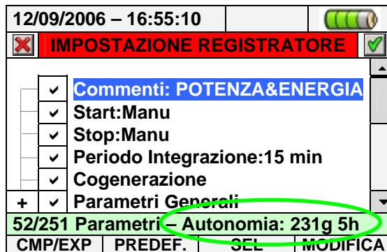
Fig. 178: Esempio di uso della memoria esterna - non presenza Compact Flash
