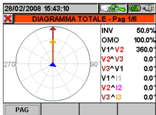
Fig. 148: Diagramma vettoriale totale in Sistema Trifase 4 fili
