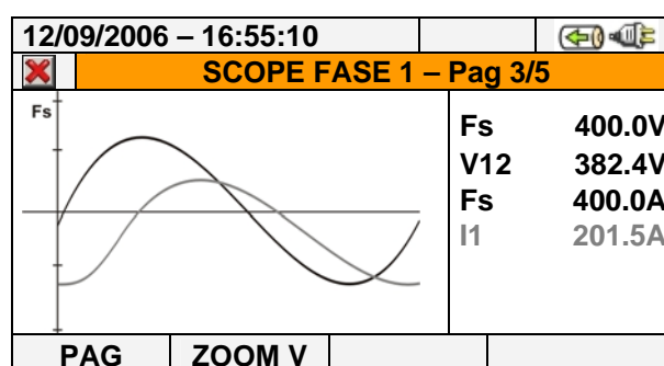
Fig. 48: Videata forme d'onda tensione e corrente fase L1 per sistemi 3-fili e ARON
