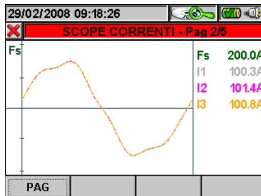
Fig. 130: Scope Correnti in Sistema Trifase 3 fili o Sistema Aron
