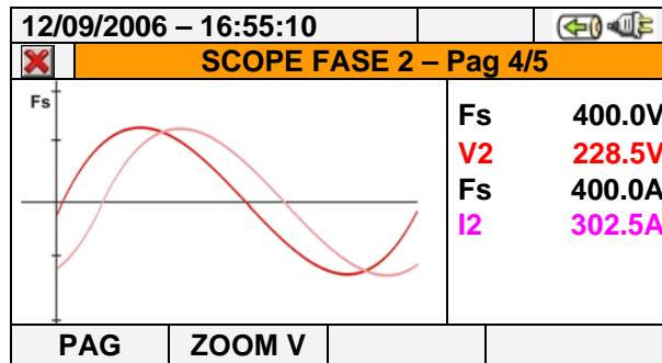
Fig. 49: Videata forme d'onda tensione e corrente fase L2 per sistemi trifase 4-fili
