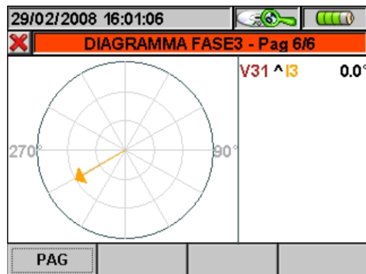
Fig. 159: Diagramma vettoriale Fase3 in Sistema Trifase 3 fili o Sistema Aron
