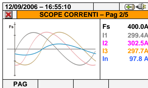
Fig. 45: Videata forme d'onda delle correnti per sistema trifase 4-fili
