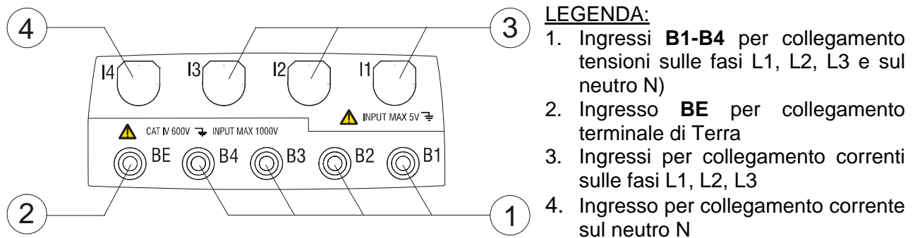
Fig. 2: Descrizione terminali di ingresso dello strumento
