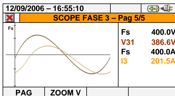
Fig. 52: Videata forme d'onda tensione e corrente fase L3 per sistemi 3-fili e ARON
