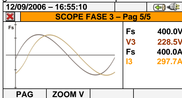
Fig. 51: Videata forme d'onda tensione e corrente fase L3 per sistemi trifase 4-fili
