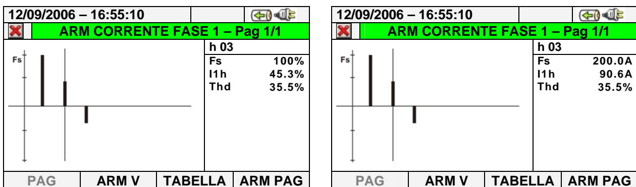
Fig. 58: Analisi armonica correnti in valore percentuale/assoluto sistemi Monofase
