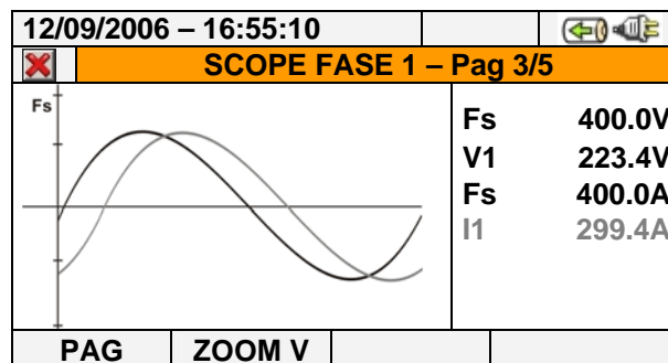
Fig. 47: Videata forme d'onda tensione e corrente fase L1 per sistemi trifase 4-fili
