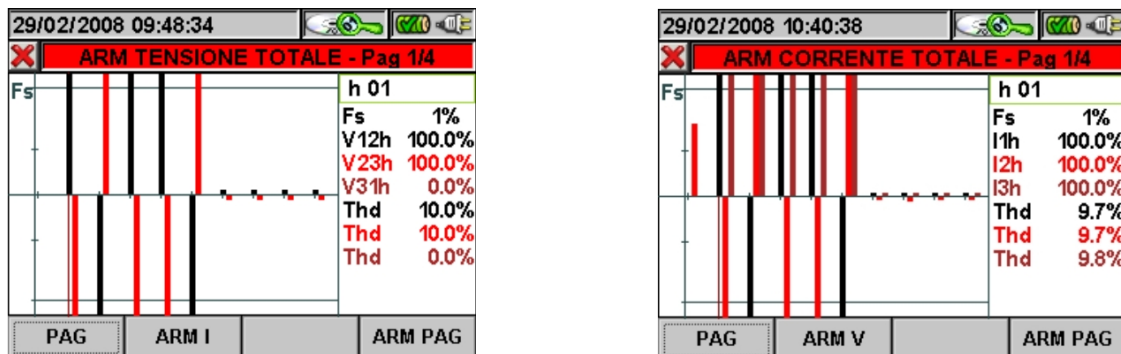
Fig. 138: Armoniche Totali in Sistema Trifase 3 fili o Sistema Aron
