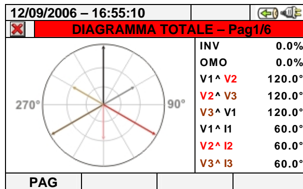
Fig. 67: Diagramma vettoriale totale per sistemi 4-fili
