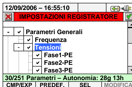
Fig. 93: Sottolivello Parametri Generali - Caso Trifase 3-fili
