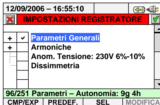
Fig. 89: Sezione Parametri Generali: parametri selezionati
