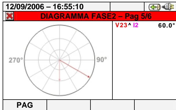
Fig. 77: Diagramma vettoriale tensione-corrente fase L2 per sistemi 3-fili e ARON
