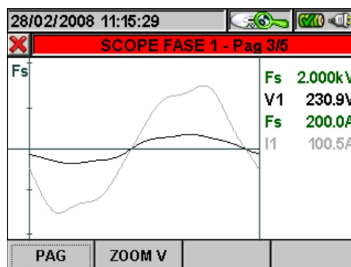
Fig. 131: Scope Fase 1 in Sistema Trifase 4 fili
