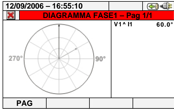
Fig. 69: Diagramma vettoriale totale per sistema Monofase
