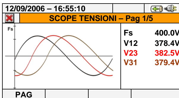
Fig. 43: Videata forme d'onda delle tensioni per sistema trifase 3-fili e ARON
