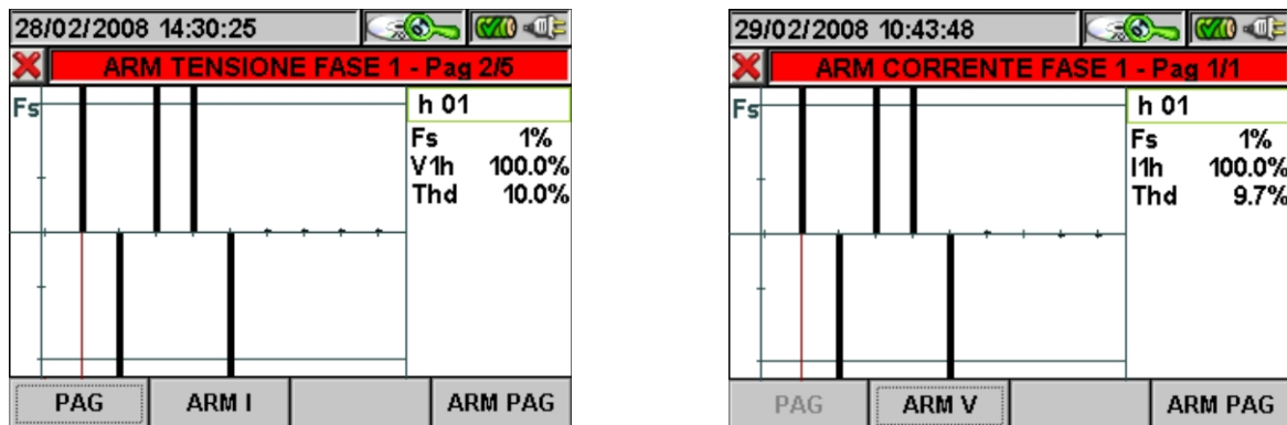
Fig. 140: Armoniche Fase1 in Sistema Trifase 4 fili
