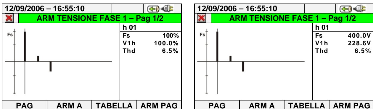
Fig. 55: Analisi armonica tensioni in valore percentuale/assoluto per sistemi Monofase
