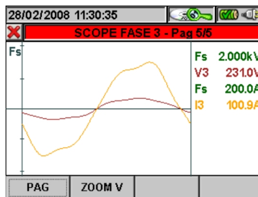
Fig. 135: Scope Fase 3 in Sistema Trifase 4 fili
