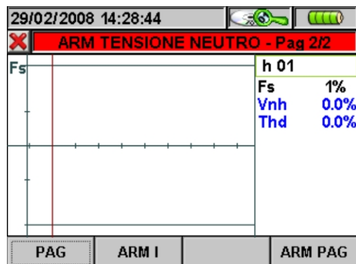
Fig. 147: Armoniche Tensione sul Neutro in Sistema Monofase
