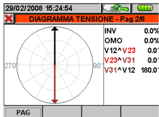
Fig. 154: Diagramma vettoriale Fase1 in Sistema Trifase 4 fili
