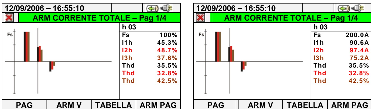
Fig. 57: Analisi armonica correnti in valore percentuale/assoluto sistemi 3-fili e ARON
