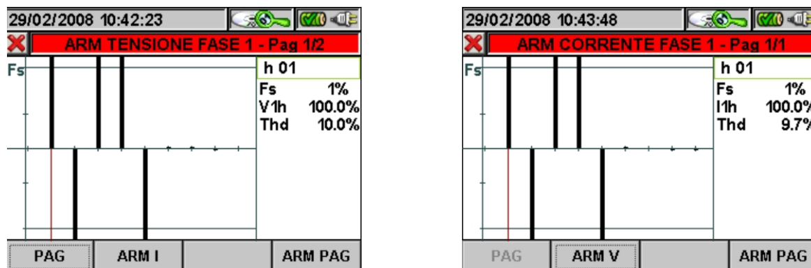
Fig. 139: Armoniche Fase 1 in Sistema Monofase
