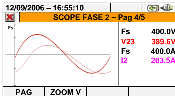
Fig. 50: Videata forme d'onda tensione e corrente fase L2 per sistemi 3-fili e ARON
