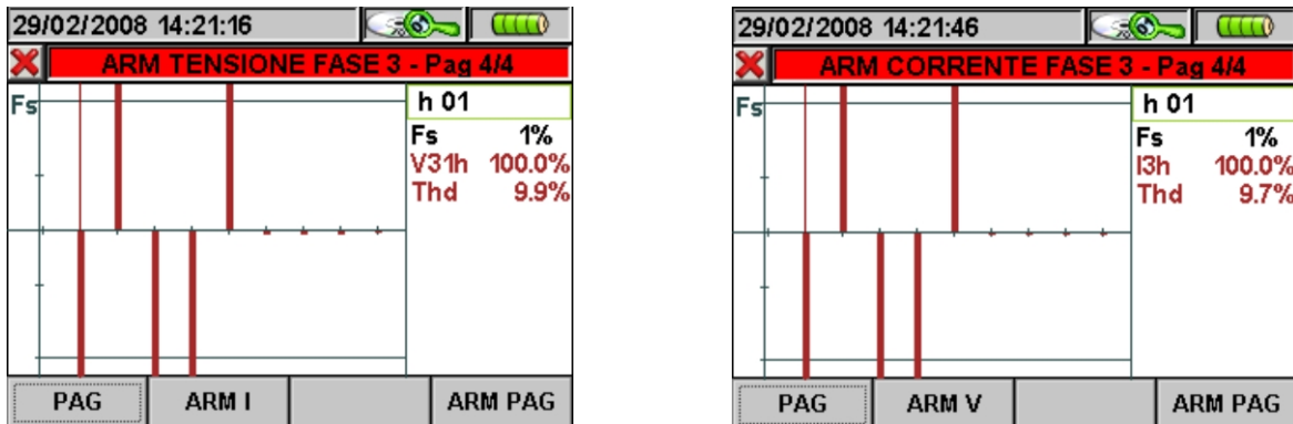
Fig. 145: Armoniche Fase3 in Sistema Trifase 3 fili o Sistema Aron
