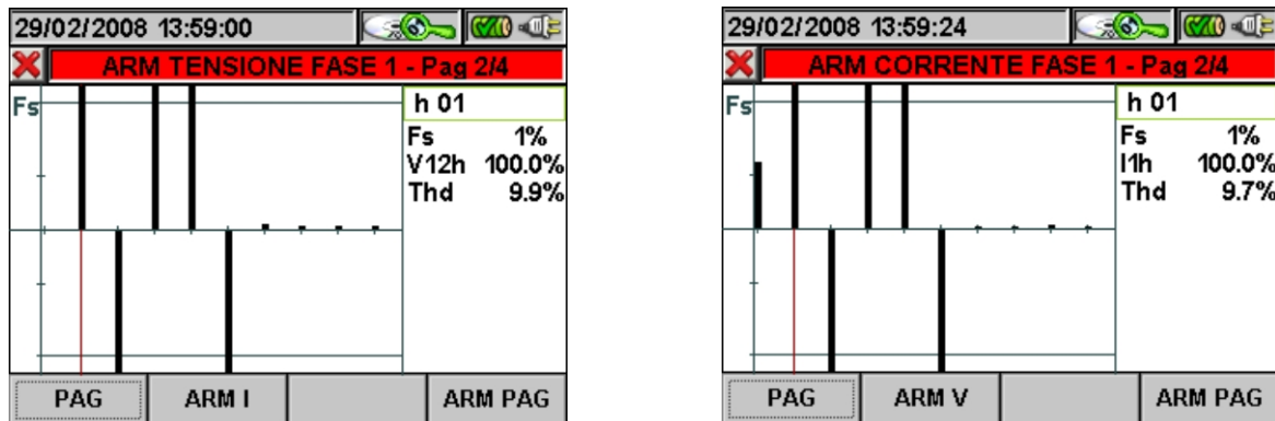
Fig. 141: Armoniche Fase1 in Sistema Trifase 3 fili o Sistema Aron
