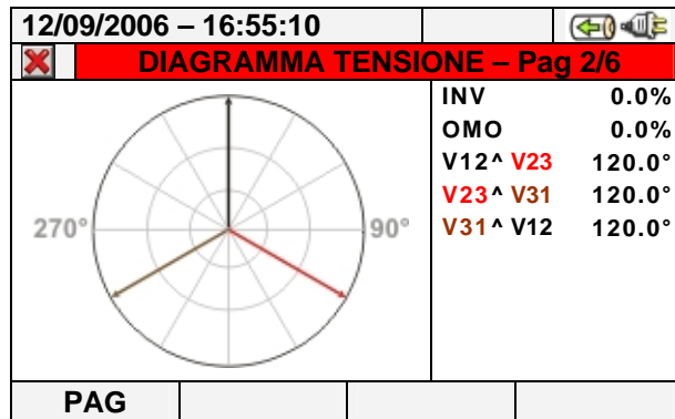
Fig. 71: Diagramma vettoriale tensioni per sistemi 3-fili e ARON
