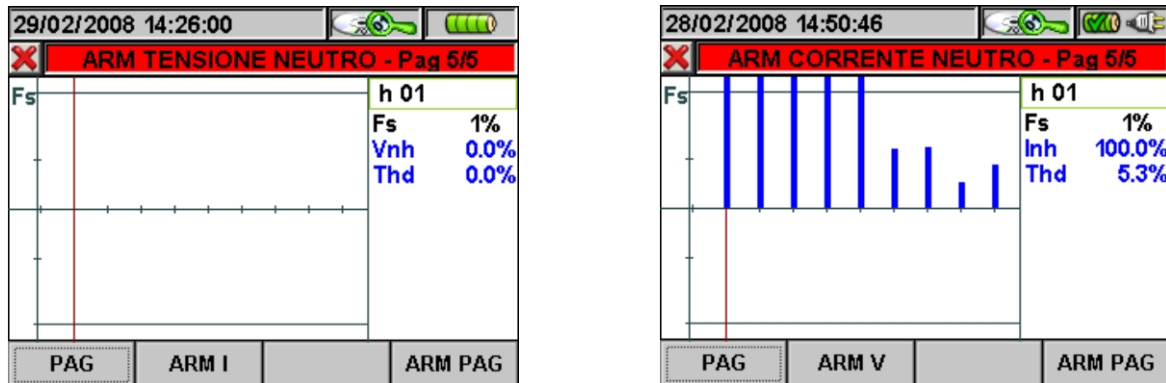
Fig. 146: Armoniche Neutro in Sistema Trifase 4 fili
