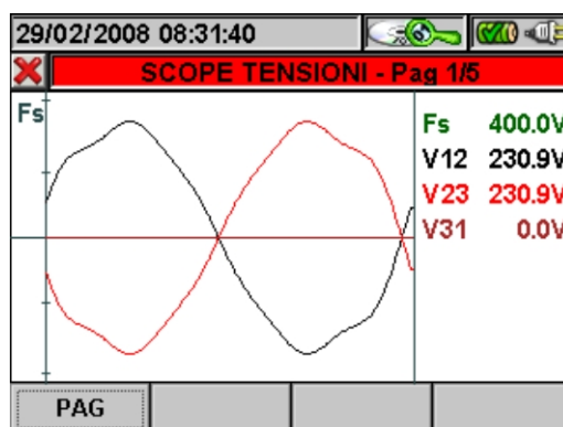
Fig. 127: Scope Tensioni in Sistema Trifase 3 fili o Sistema Aron
