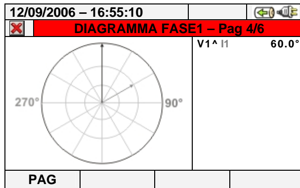
Fig. 73: Diagramma vettoriale tensione-corrente fase L1 per sistemi 4-fili
