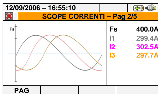
Fig. 46: Videata forme d'onda delle correnti per sistemi trifase 3-fili e ARON
