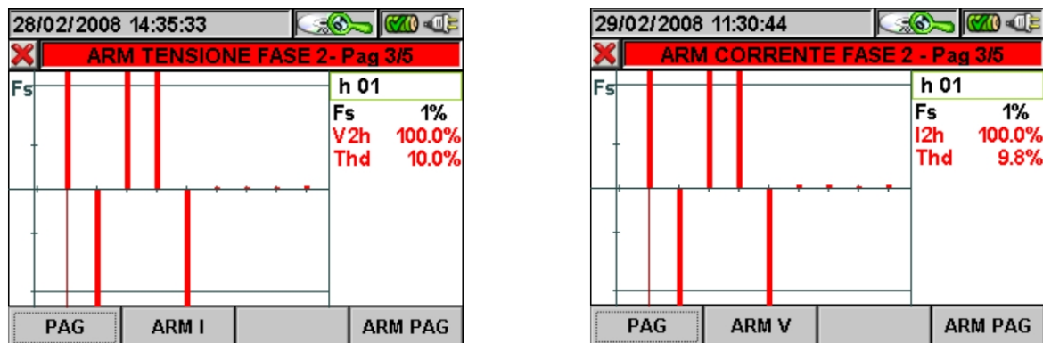
Fig. 142: Armoniche Fase2 in Sistema Trifase 4 fili
