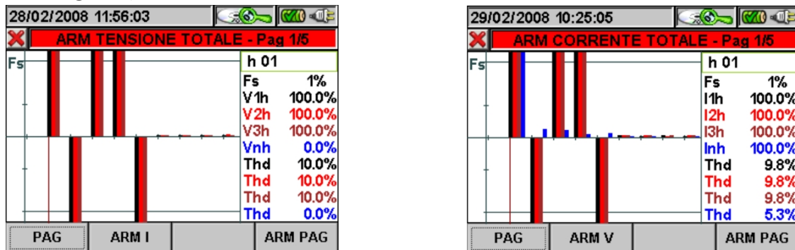
Fig. 137: Armoniche Totali in Sistema Trifase 4 fili
