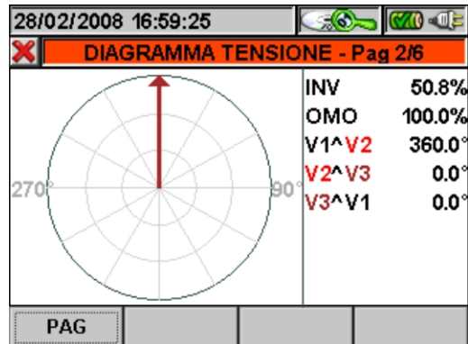
Fig. 153: Diagramma vettoriale Correnti in Sistema Trifase 4 fili, Sistema Trifase 3 fili o Sistema Aron
