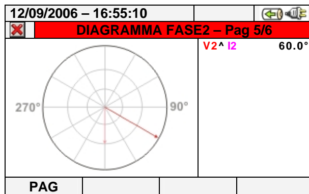
Fig. 74: Diagramma vettoriale tensione-corrente fase L2 per sistemi 4-fili
