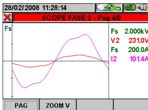
Fig. 133: Scope Fase 2 in Sistema Trifase 4 fili
