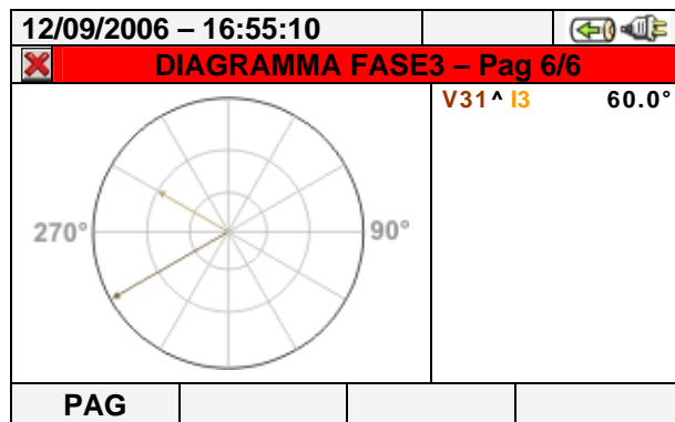
Fig. 78: Diagramma vettoriale tensione-corrente fase L3 per sistemi 3-fili e ARON
