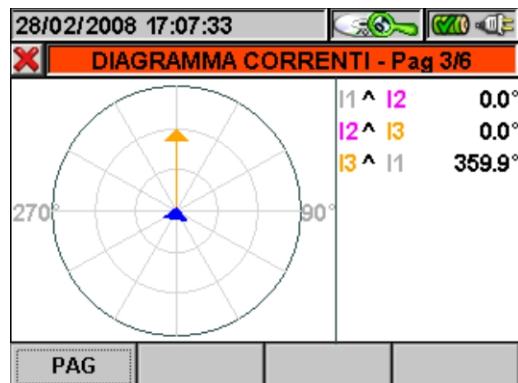
Fig. 155: Diagramma vettoriale Fase1 in Sistema Trifase 3 fili o Sistema Aron
