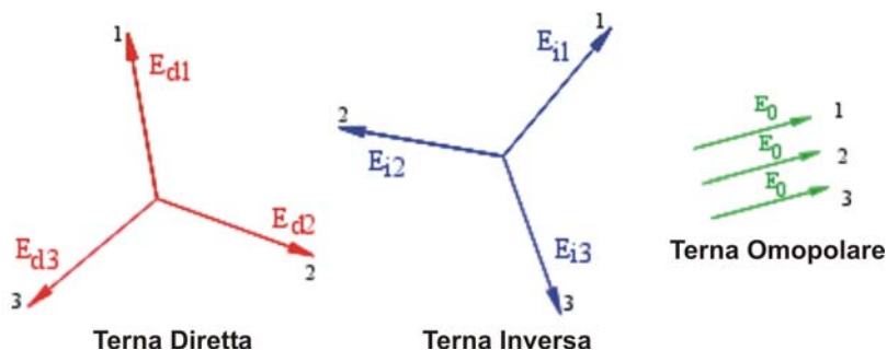
Fig. 189: Scomposizione di una terna di vettori
