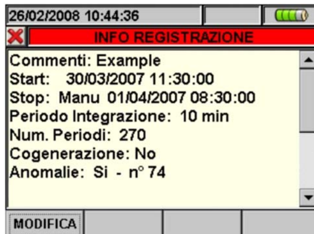
Fig. 115: Info Registrazione
