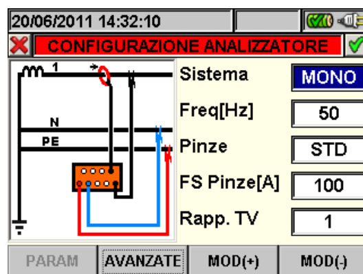
Fig. 83: Videata configurazione analizzatore per sistema Monofase
