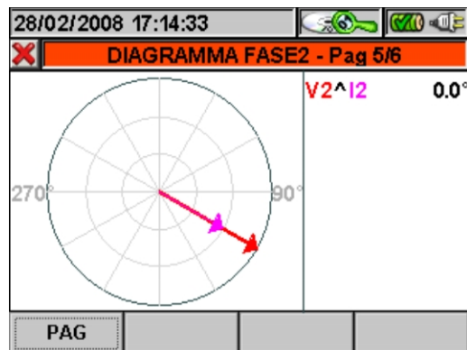
Fig. 157: Diagramma vettoriale Fase2 in Sistema Trifase 3 fili o Sistema Aron
