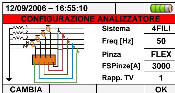
Fig. 6: Esempio di configurazione analizzatore
