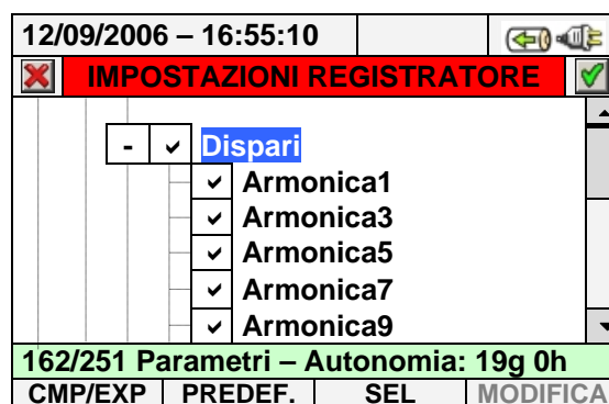
Fig. 96: Sottolivello Armoniche – selezione Armoniche Dispari
