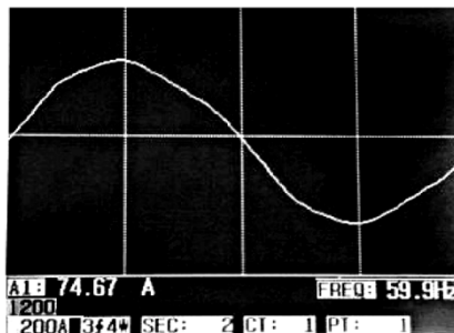
Forme d'Onda - Schermata 2
