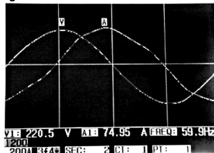
Figura 5-9c: Forme d'Onda - Schermata 3
