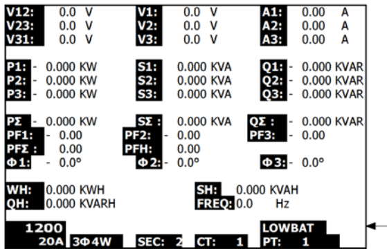
Indicazione Batteria Scarica
