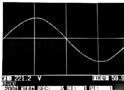
Forme d'Onda - Schermata 2
