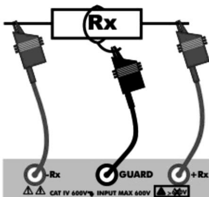
Fig. 4: Connessione dello strumento
