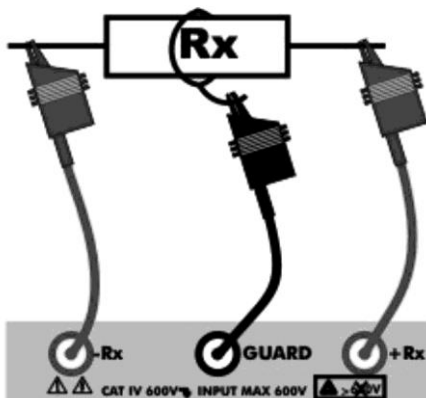
Fig. 6: Connessione dello strumento
