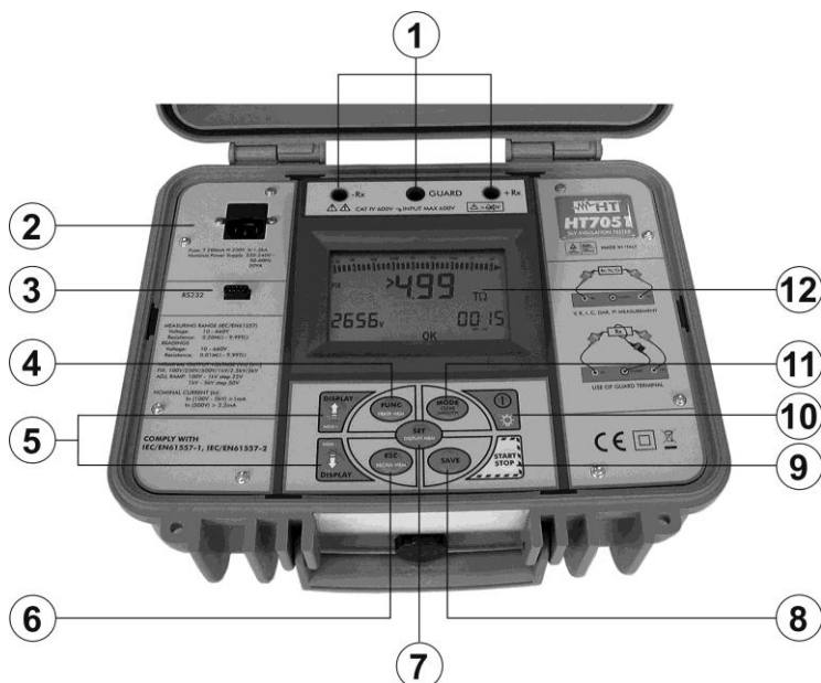
Fig. 1: Descrizione dello strumento
