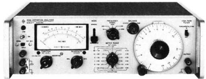
HP 334A
