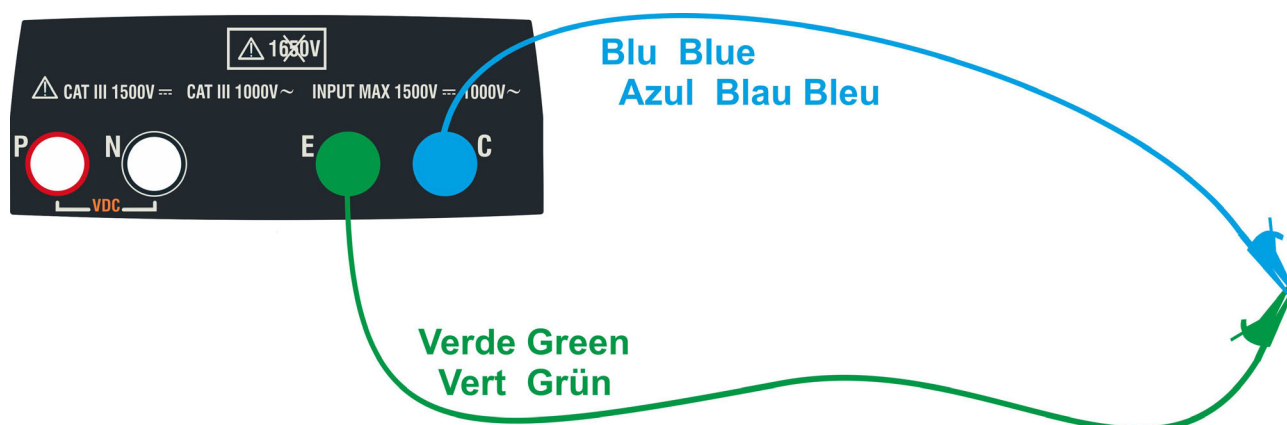
Fig. 4: Compensazione della resistenza dei cavi di misura
