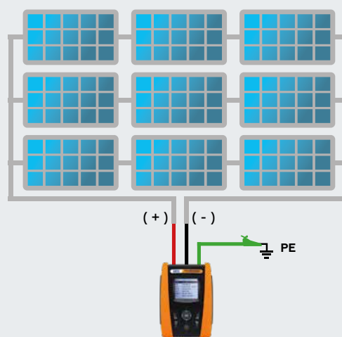
Isolamento modo DUAL Campo FV non collegato a terra
