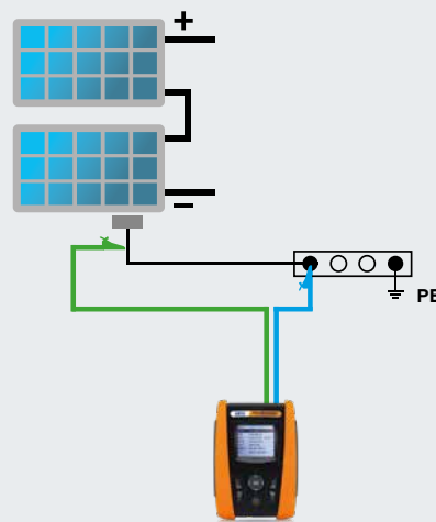
FUNZIONE RPE Schema di collegamento
