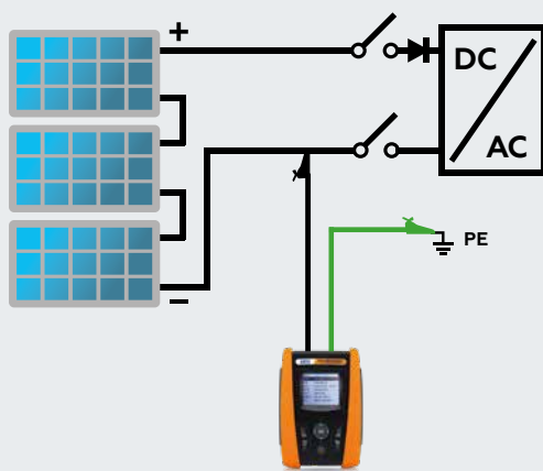
Isolamento modo TIMER Schema di collegamento
