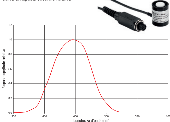
Curva di risposta spettrale relativa
