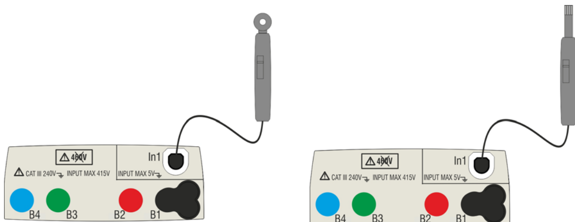
Fig. 31: Misura parametri ambientali con sonde esterne
