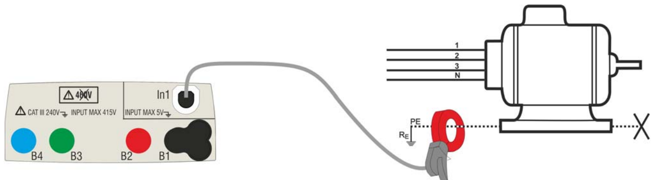
Fig. 25: Misurazione diretta della corrente di dispersione in impianti trifase
