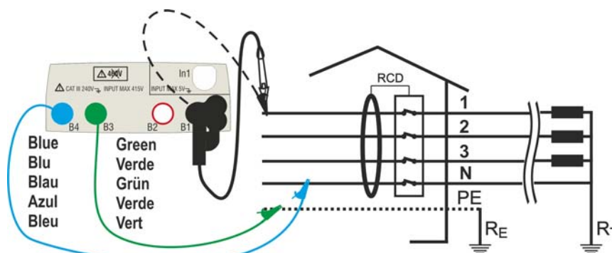
Fig. 12: Collegamento in sistema trifase 400V + N + PE con cavi singoli e puntale remoto
