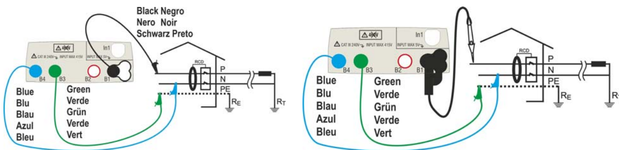
Fig. 11: Collegamento in sistema monofase 230V con cavi singoli e puntale remoto
