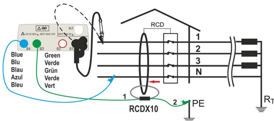
Fig. 15: Collegamento a RCD con toroide separato con accessorio opzionale RCDX10
