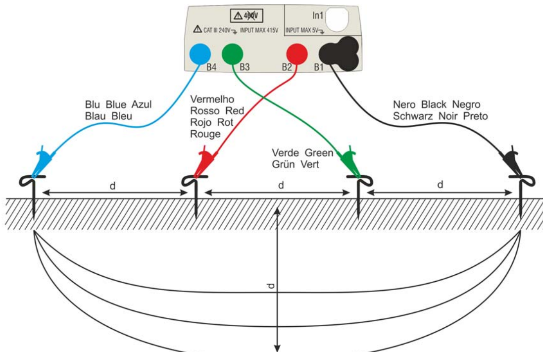
Fig. 29: Misura della resistività del terreno
