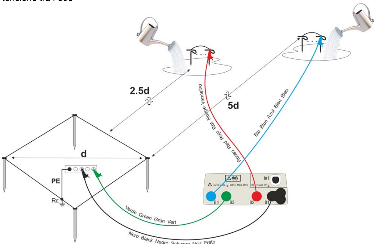
Fig. 39: Misura di terra per reti di terra di piccole dimensioni
