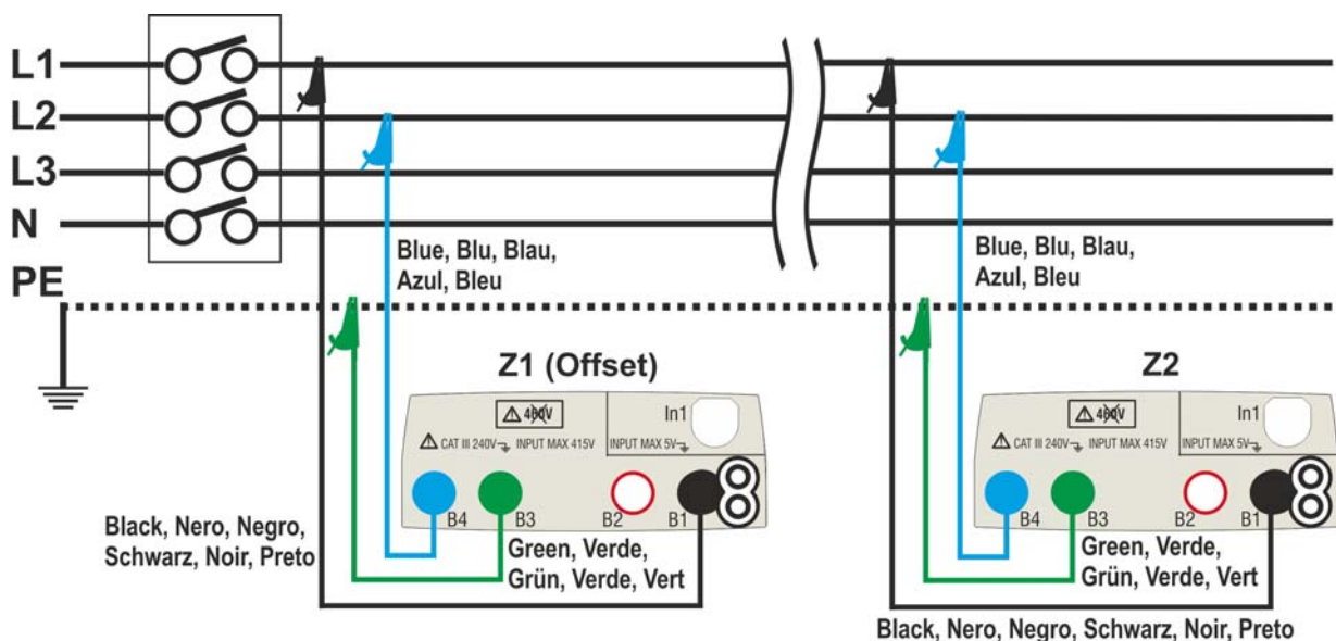
Fig. 33: Collegamento strumento per misura caduta di tensione in modo L-L
