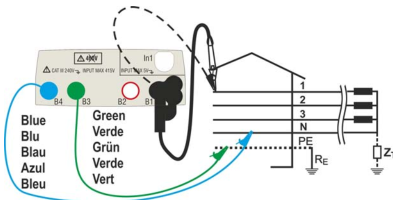
Fig. 21: Misura P-PE in sistemi IT con cavi singoli e puntale remoto
