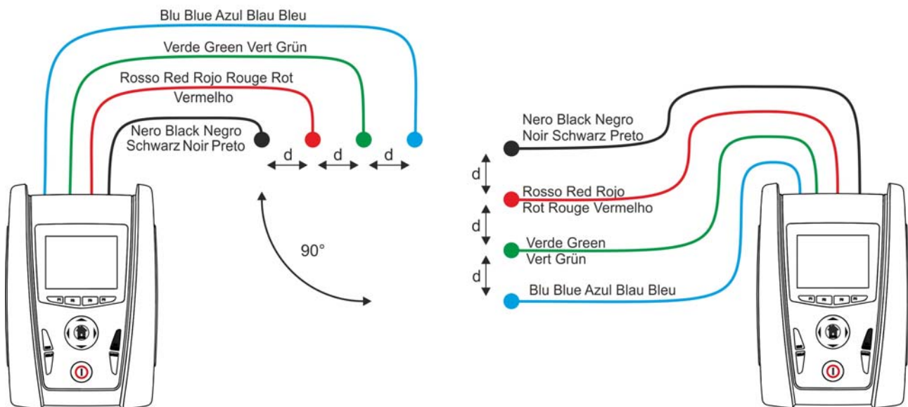
Fig. 41: Misura della resistività del terreno
