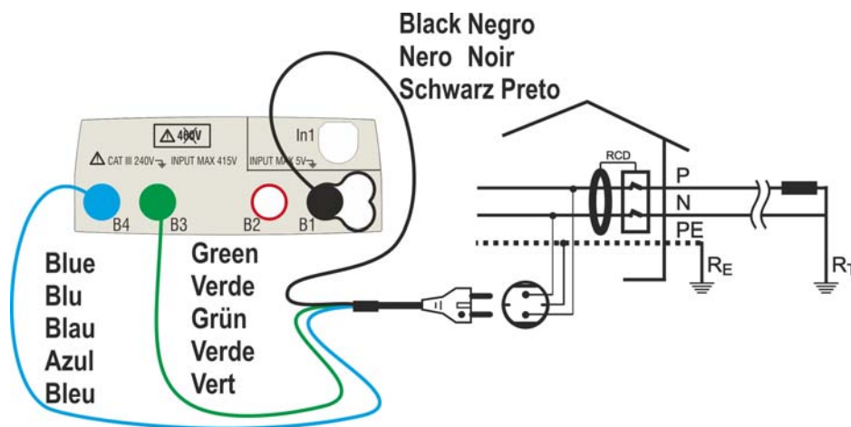
Fig. 10: Collegamento in sistema monofase 230V tramite spina shuko
