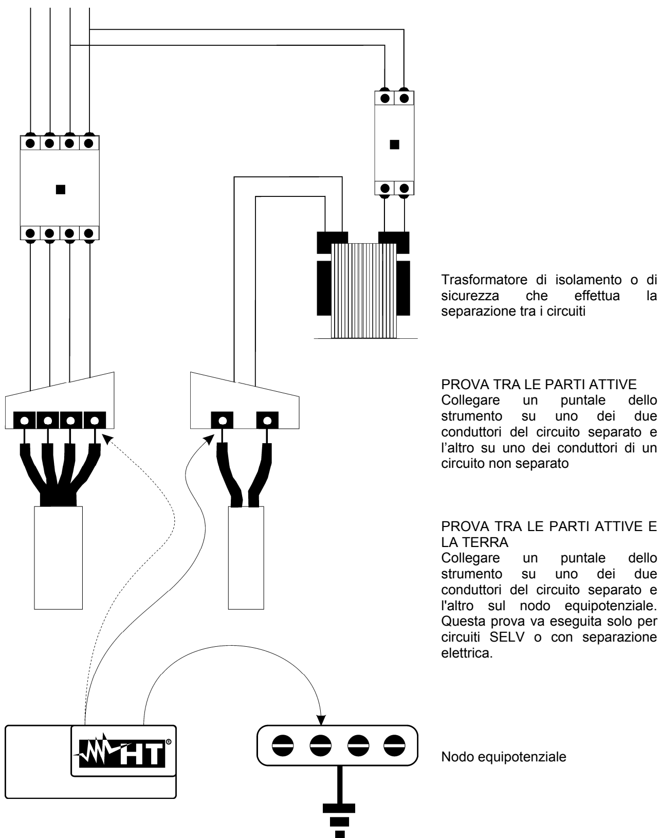
Fig. 37: Misure di separazione tra circuiti in un impianto
