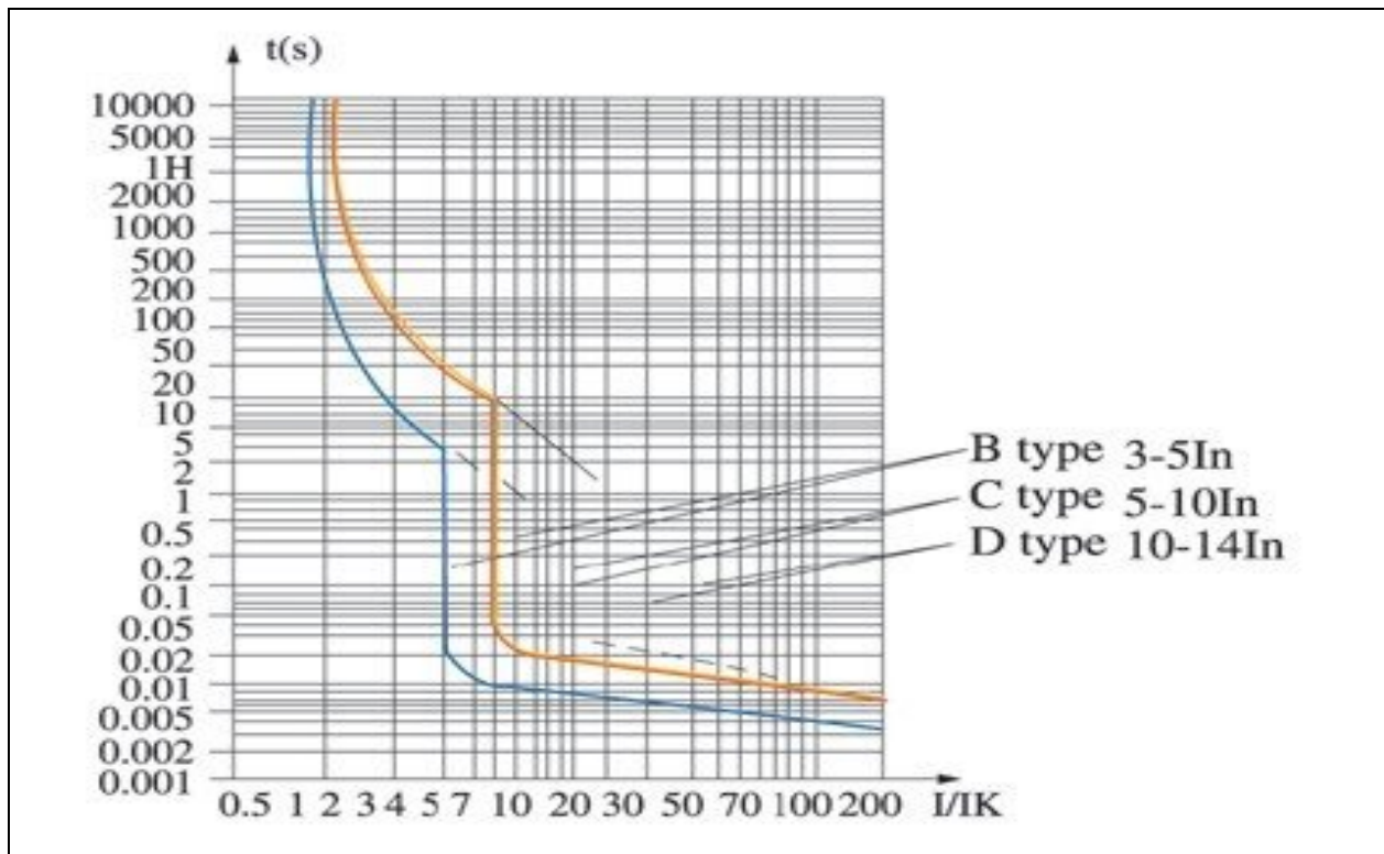
Fig. 38: Esempio di curve di intervento protezioni magnetotermiche (MCB)
