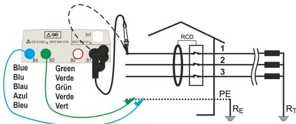
Fig. 14: Collegamento in sistema trifase 400V+ PE (no N) con cavi singoli e puntale remoto ( no RCD tipo B )
