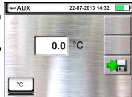
Fig. 31: Misura parametri ambientali con sonde esterne
