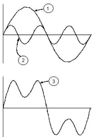
Fig. 43: Effetto della sovrapposizione di due frequenze multiple l'una dell'altra
