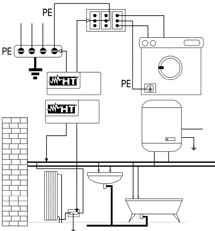
Fig. 36: Esempi di misure di continuità dei conduttori
