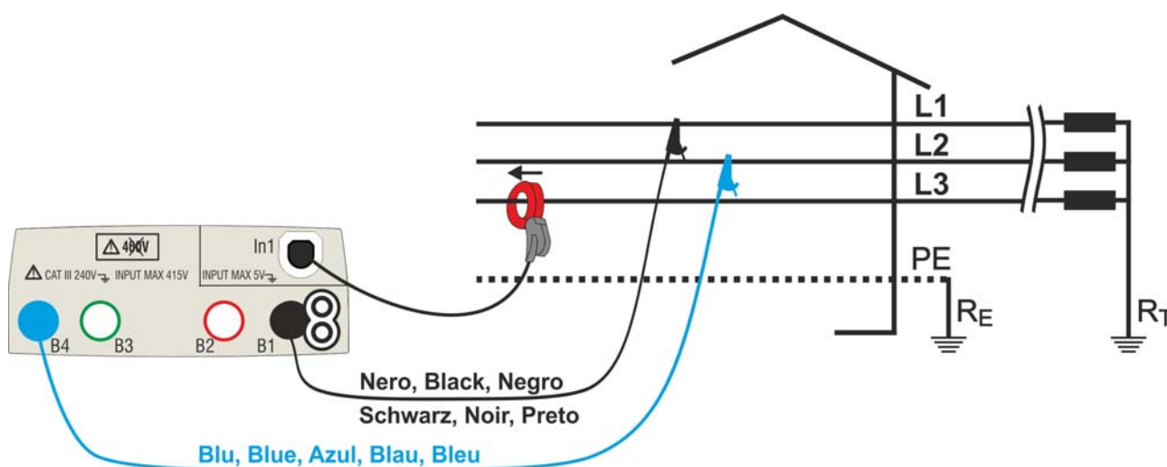
Fig. 35: Collegamento per misura su impianto Trifase equilibrato
