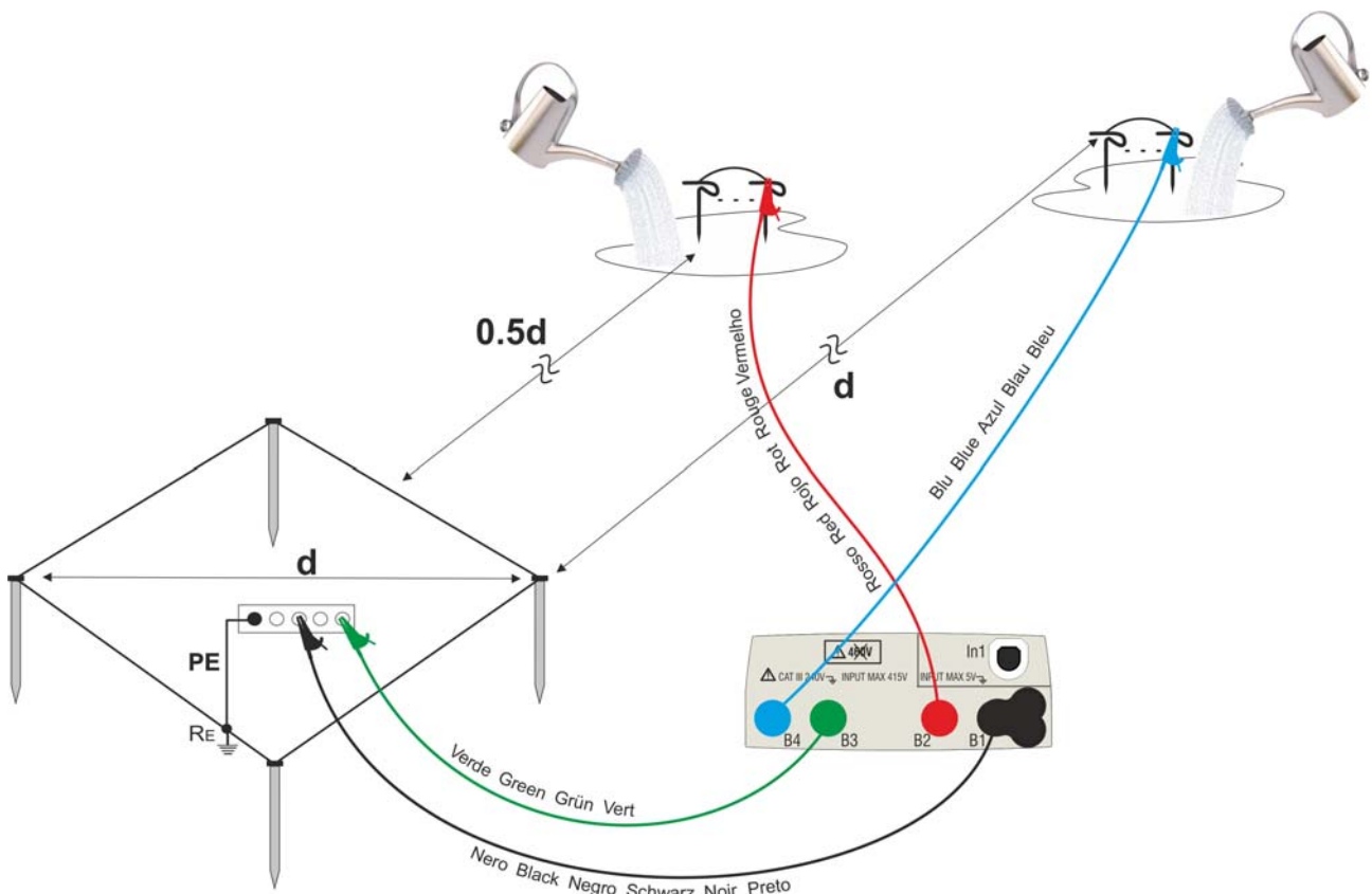
Fig. 40: Misura di terra per reti di terra di grandi dimensioni
