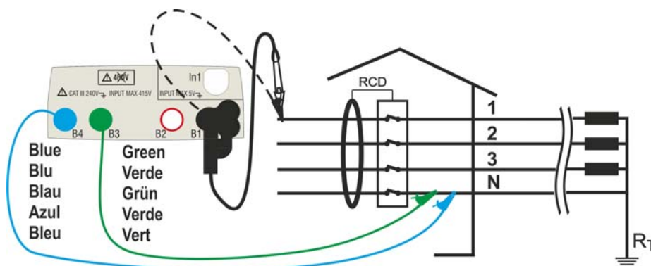
Fig. 13: Collegamento 400V+ N (no PE) con cavi e puntale remoto ( no RCD tipo B )
