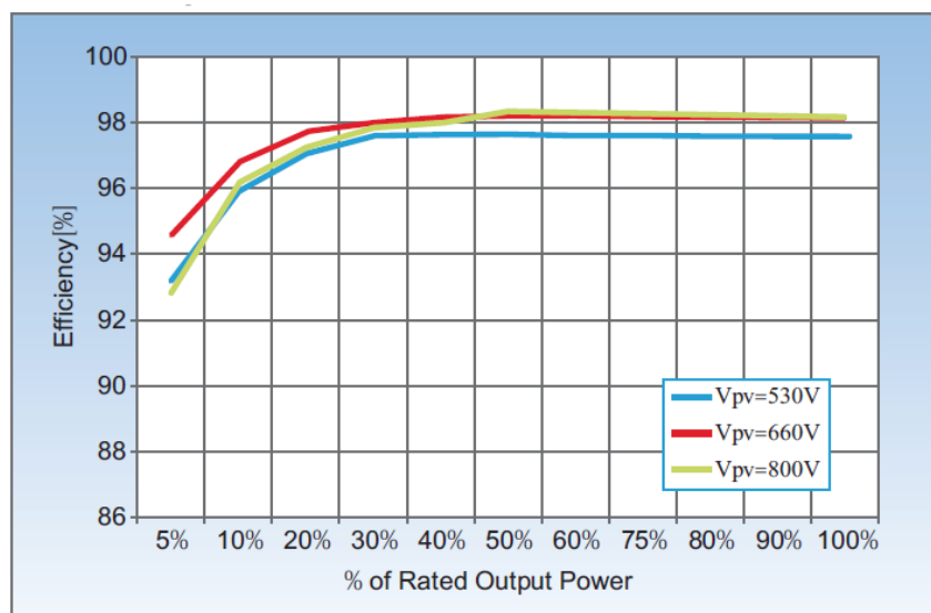
Figura 8 – Curva di efficienza per un inverter Azzurro ZCS della famiglia 50K-70 TL
