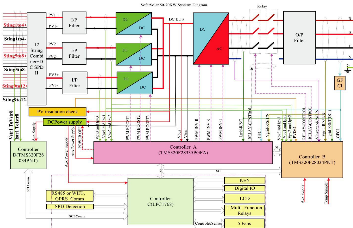
Figura 7 - Schema di funzionamento a blocchi degli inverter della serie 50K-70K TL
