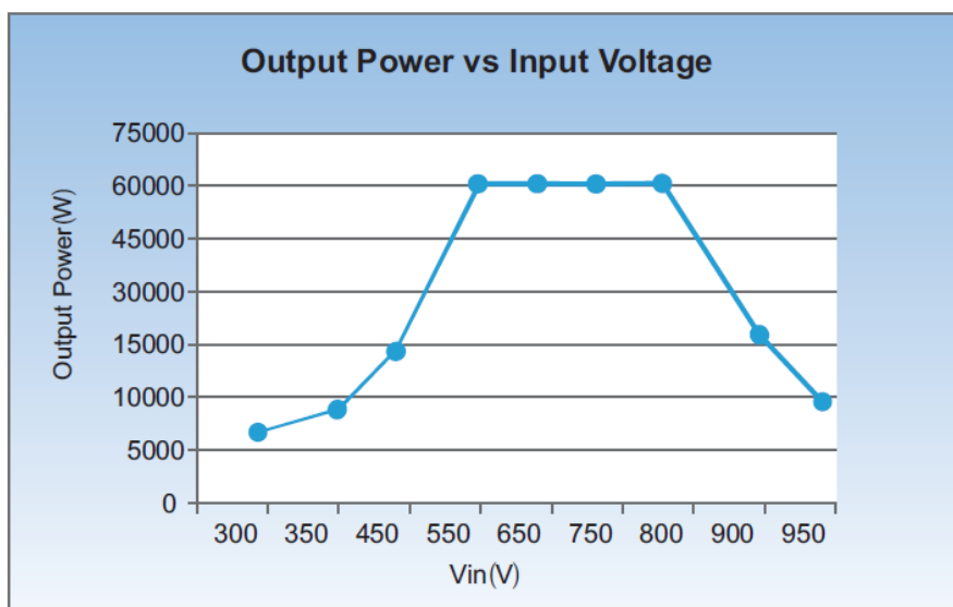
Figura 9 - Curva di derating della tensione in ingresso per un inverter Azzurro ZCS della famiglia 50K-70 TL
