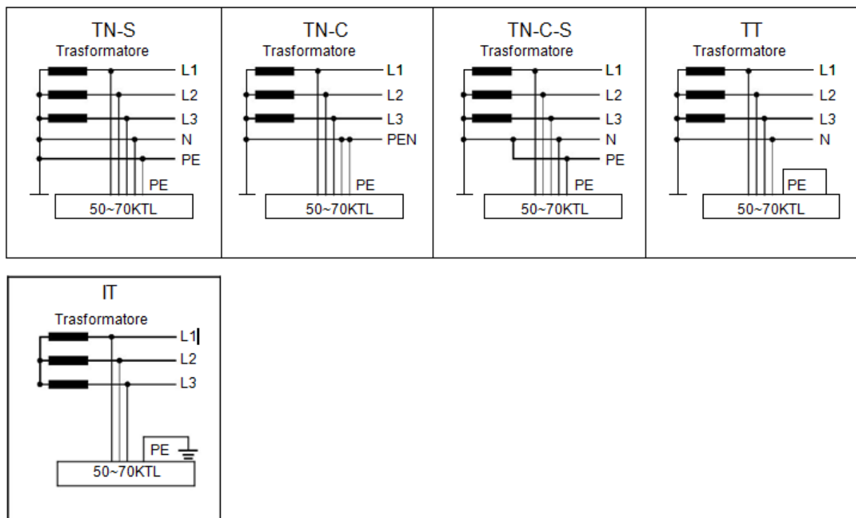
Figura 3 - Schemi elettrici dei tipi di rete su cui poter installare gli inverter 50K-70K TL
