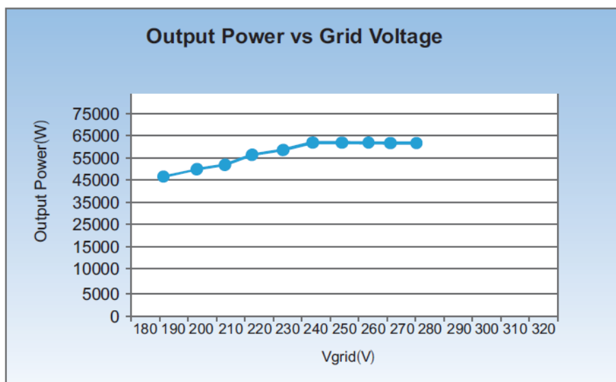
Figura 10 - Curva di derating della tensione in uscita per un inverter Azzurro ZCS della famiglia 50K-70 TL
