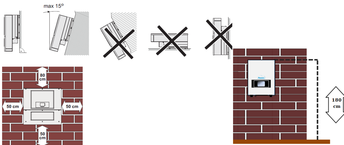
Figura 12 – Requisiti di installazione per un singolo inverter
