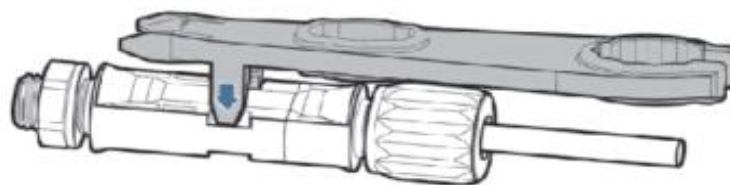
Figura 25- Rimozione del connettore DC
