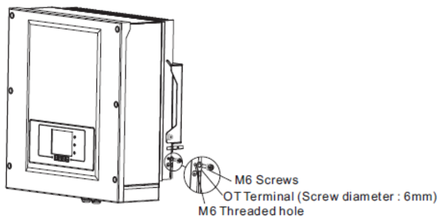
Figura 12 - Collegamento del terminale di terra
