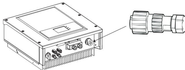
Figura 25 - Connessione dei cavi AC di uscita (4)
