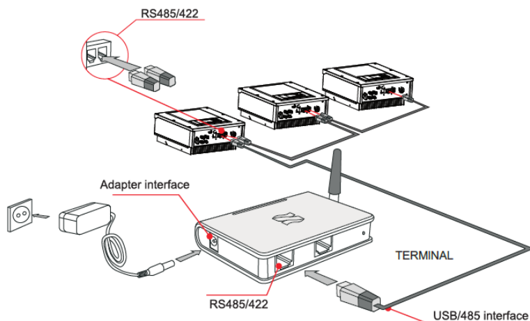
Figura 34 - Installazione con più inverter
