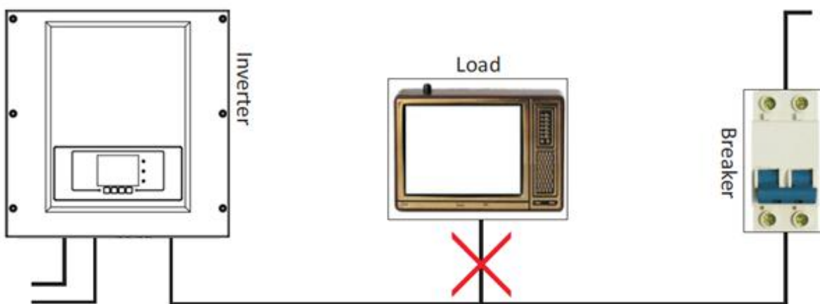
Figura 21 - Non è consentito connettere carichi tra l'inverter e il sezionatore
