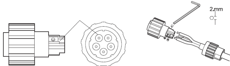
Figura 24 - Connessione dei cavi AC di uscita (3)
