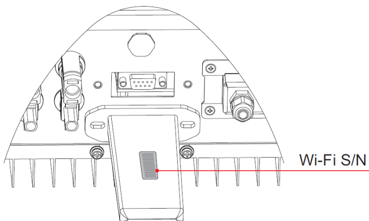
Figura 31 - Installazione del modulo wifi/GPRS
