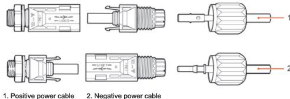
Figura 18 - Connessione dei cavi di potenza DC in ingresso (2)
