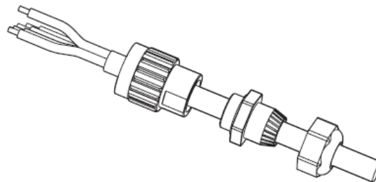
Figura 23 - Connessione dei cavi AC di uscita (2)
