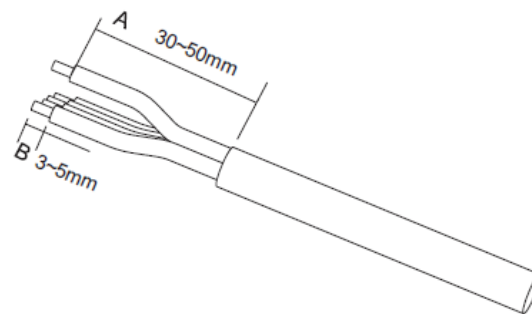
Figura 22 - Connessione dei cavi AC di uscita (1)
