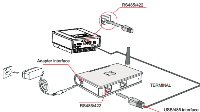
Figura 33 - Installazione con un solo inverter
