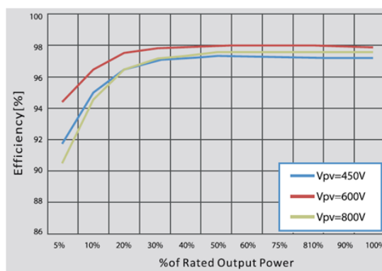
Figura 6 – Curva di efficienza per un inverter Azzurro ZCS 11KTL-X
