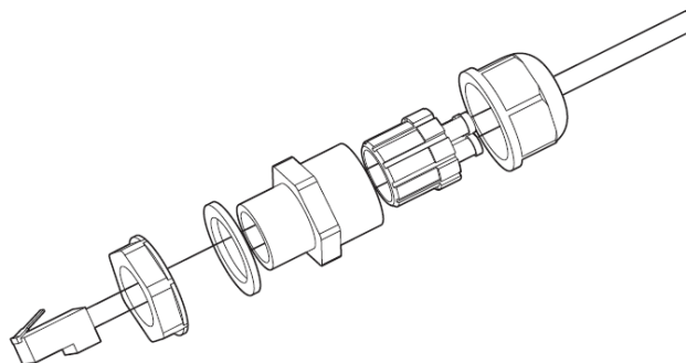
Figura 28 - Montaggio del connettore di comunicazione
