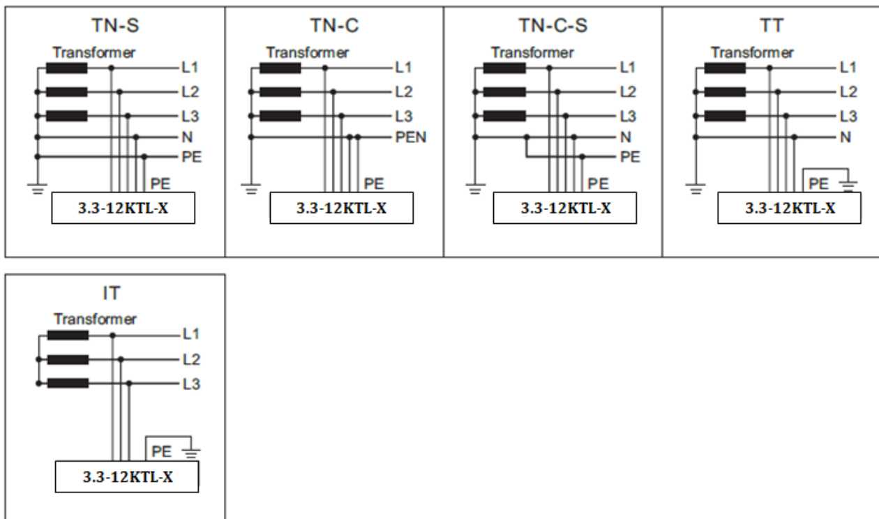
Figura 3 - Schemi elettrici dei tipi di rete su cui poter installare gli inverter 3.3K-12KTL-X
