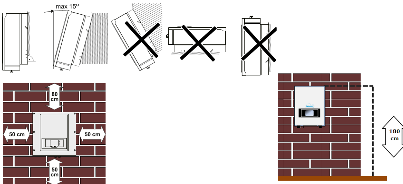
Figura 8 - Requisiti di installazione per un singolo inverter
