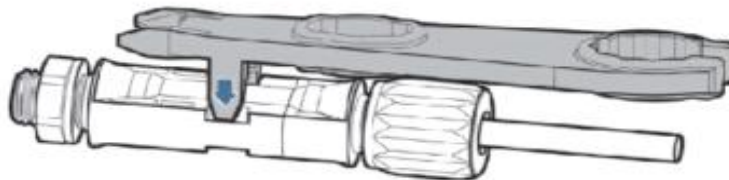
Figura 20- Rimozione del connettore DC
