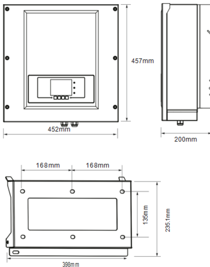
Figura 4 - Vista frontale, laterale e posteriore dell'inverter e della staffa
