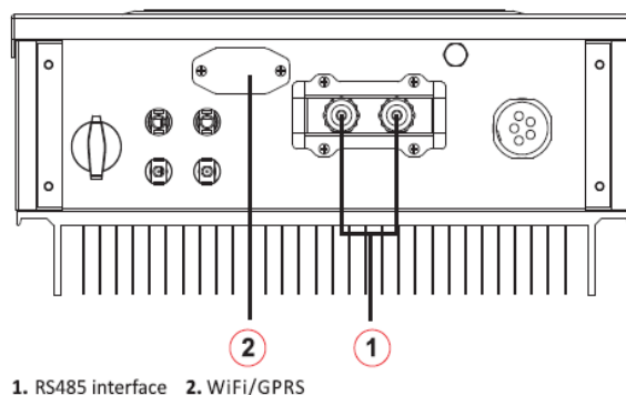
Figura 26 - Vista inferiore dell'inverter con interfaccia RS485 (1) e Wifi (2)
