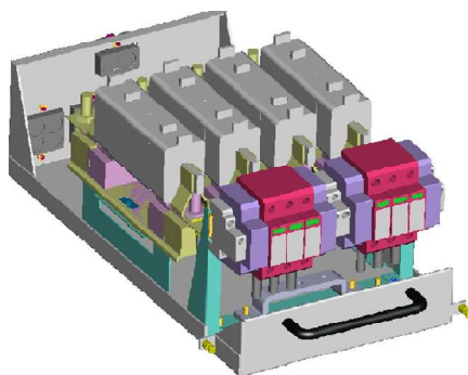
Figura 17-3: Cassetto DC
