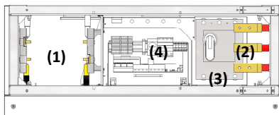
Figura 10-11: Composizione Zona ACBOX (versioni con potenza \geq 275\text{kW} o senza Trasformatore)
