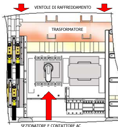
Figura 5-6: Ingresso Cavi AC (versioni con Trasformatore \leq 220\text{kW} )
