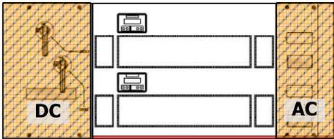
Figura 16-5: Pannellature da rimuovere accesso Fusibili DC e AC.
