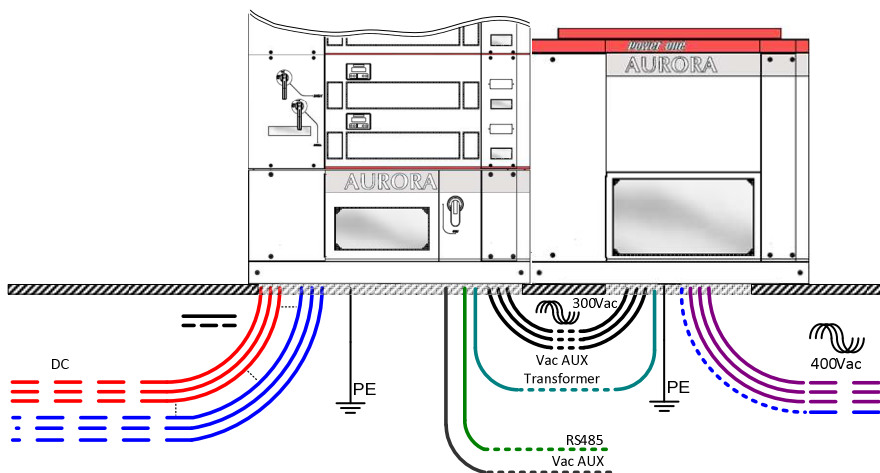
Figura 10-12: Uscita cavi sotto l'inverter (versioni \geq 275\text{kW} )
