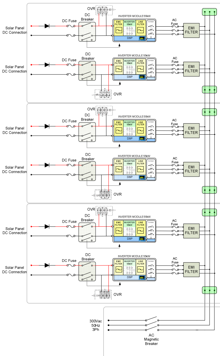
Figura 4-7: Schema elettrico di massima del PVI-XXX.0(-TL) senza Trasformatore (per tutte le versioni)
