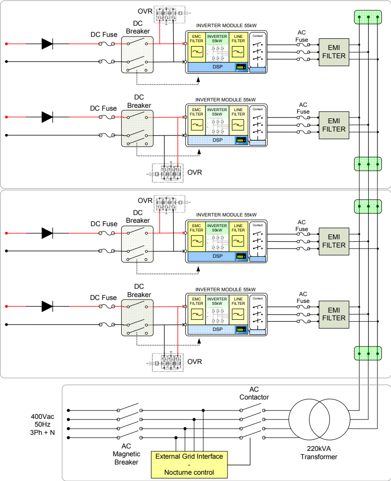
Figura 4-5: Schema elettrico di massima del PVI-XXX.0 con Trasformatore a bordo (≤220kW)
