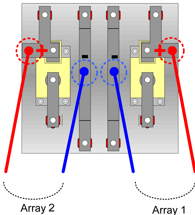
Figura 11-2- Configurazione Multi-Master
