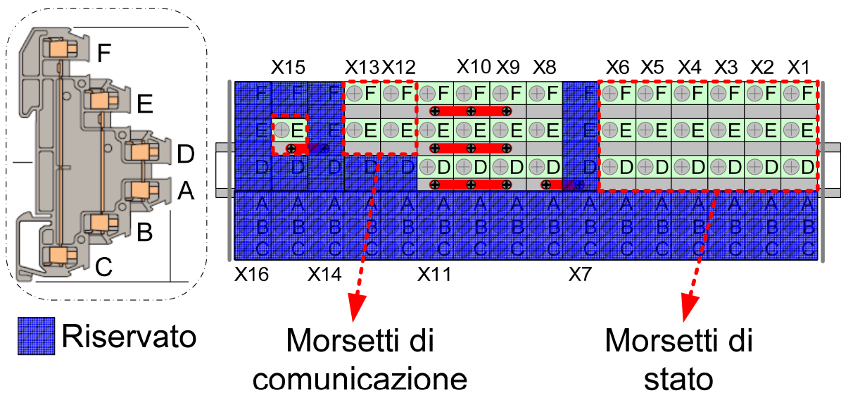
Figura 11-8: Morsettieria interna zona ACBOX
