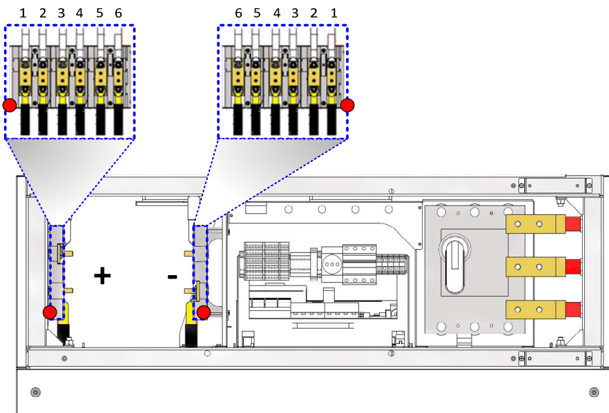
Figura 11-1: Collegamento dei cavi DC (versioni con potenza \geq 275\text{kW} o senza Trasformatore)
