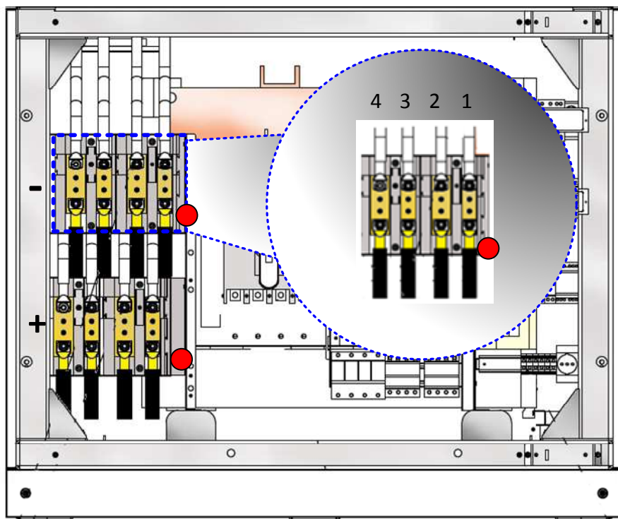
Figura 11-2: Collegamento dei cavi DC (versioni con Trasformatore \leq 220\text{kW} )
