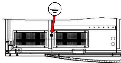
Figura 11-4: Collegamento del cavo di Terra di protezione (PE) per ACBOX con Trasformatore
