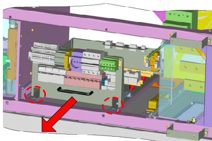
Figura 17-4: Viti di tenuta cassetto AC
