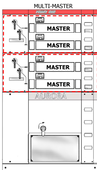
Figura 6-2: Composizione PVI-220.0 (Multi-Master)
