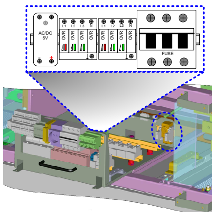
Figura 17-5: Posizione di manutenzione del cassetto AC
