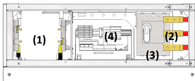
Figura 10-11: Composizione Zona ACBOX (versioni con potenza \geq 275\text{kW} o senza Trasformatore)
