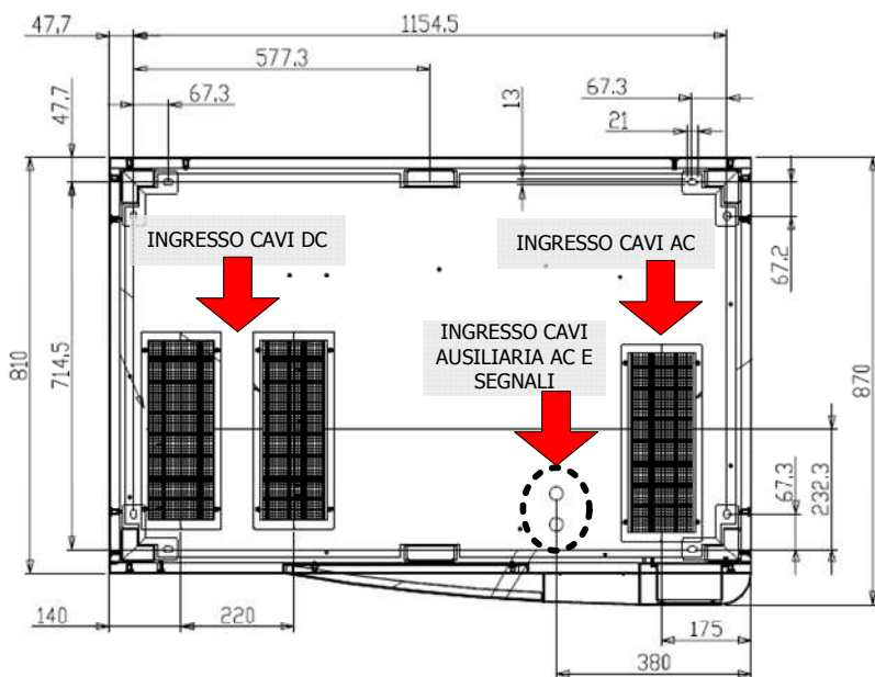
Figura 10-3: Fori passaggio cavi per sistemi \geq 275\text{kW} e tutti i modelli senza Trasformatore
