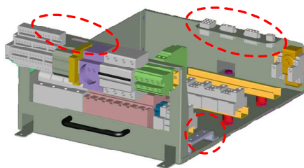
Figura 17-6: Cassetto AC
