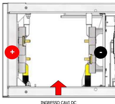
Figura 5-10: Ingresso Cavi DC (versioni con potenza \geq 275\text{kW} o senza Trasformatore)
