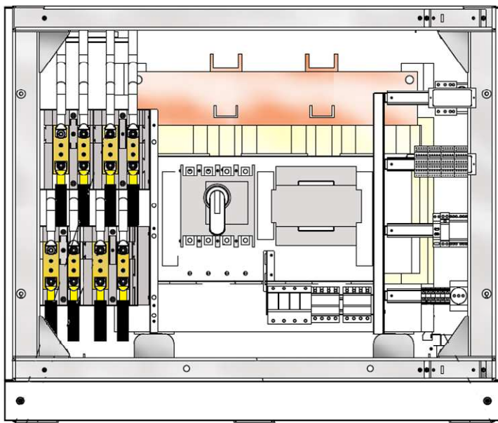
Figura 5-3: Vista generale ACBOX (A) (versioni con Trasformatore \leq 220\text{kW} )
