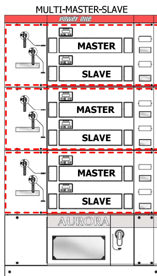
Figura 6-3: Composizione PVI-330.0(-TL) (Multi-Master-Slave)
