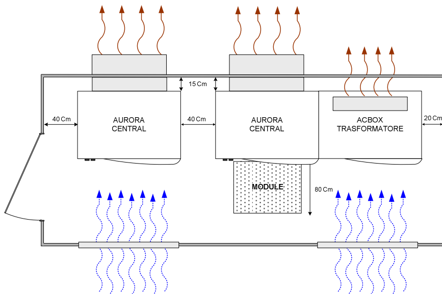
Figura 10-8: Esempio di installazione
