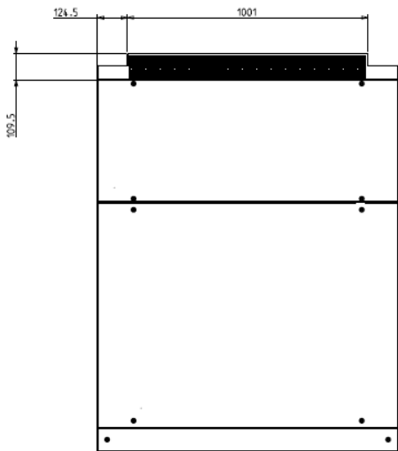
Figura 10-6: Cappa uscita aria calda per versioni fino a 110kW
