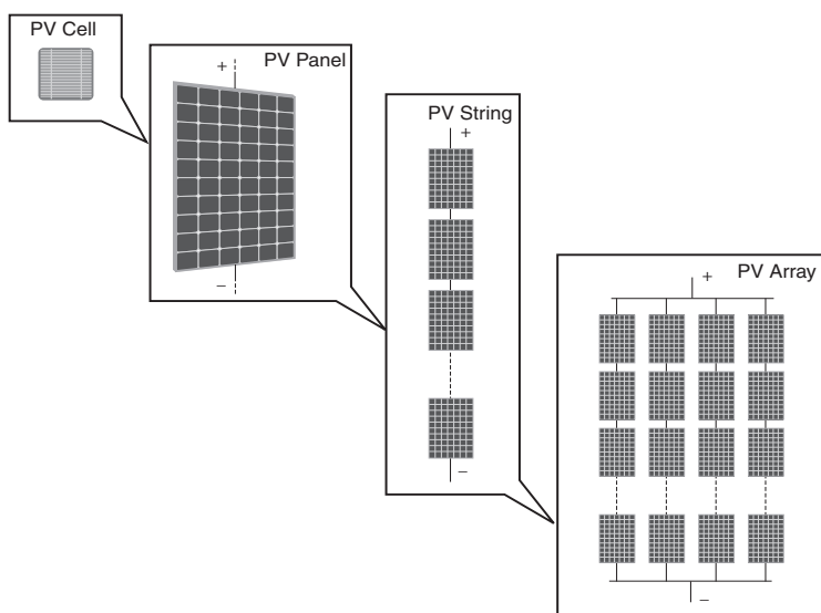
Figura 3-1: Composizione Array
