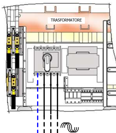
Figura 11-6: Collegamento cavi AC di potenza (versioni con potenza \leq 220\text{kW} )
