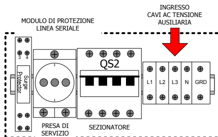
Figura 11-7: Morsetti di collegamento rete AC ausiliaria e relativo interruttore magnetotermico (versioni con potenza \geq 275\text{kW} o senza Trasformatore)
