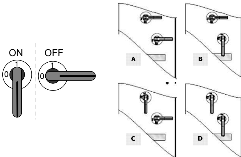
Figura 6-8: Possibili posizioni degli interruttori
