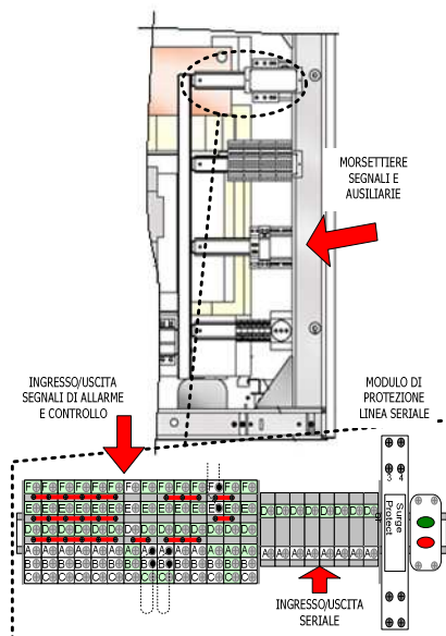
Figura 5-8: Ingresso/Uscite segnali (versioni con Trasformatore \leq 220\text{kW} )
