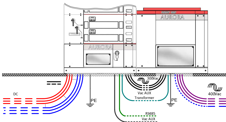
Figura 10-12: Uscita cavi sotto l'inverter (versioni \geq 275\text{kW} )
