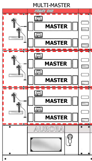
Figura 6-1: Composizione PVI-330.0-TL (Multi-Master)
