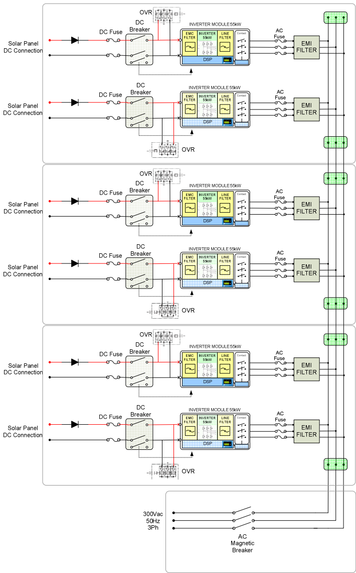
Figura 4-7: Schema elettrico di massima del PVI-XXX.0(-TL) senza Trasformatore (per tutte le versioni)
