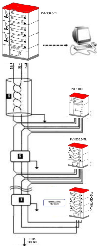
Figura 8-4: Tipologia di connessione dei PVI-XXX.0(-TL)
