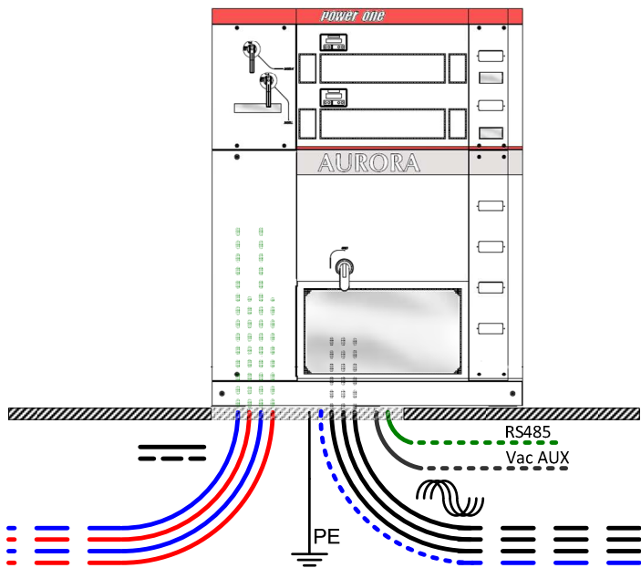
Figura 10-14: Uscita cavi sotto l'inverter (versioni ≤220kW)
