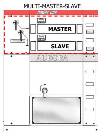
Figura 6-4: Composizione PVI-110.0 (Master-Slave)
