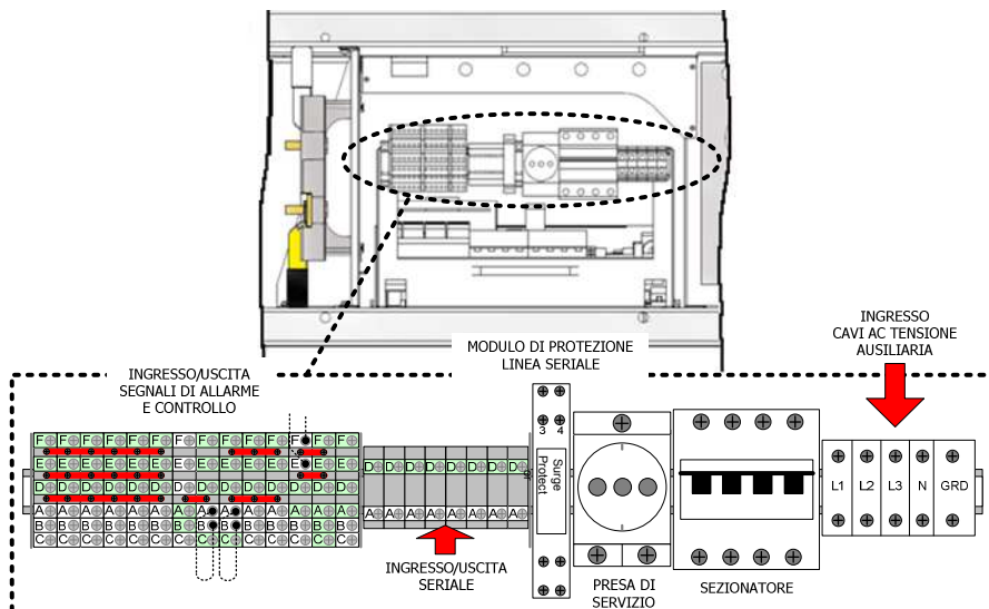
Figura 5-12: Ingresso/Uscite segnali (versioni con potenza \geq 275\text{kW} o senza Trasformatore)
