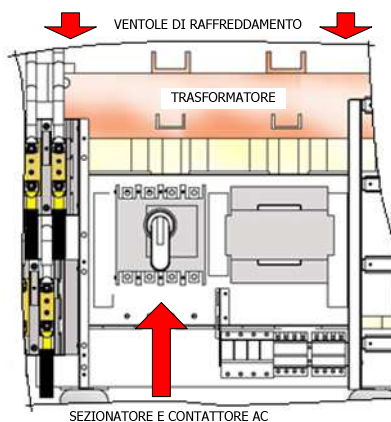
Figura 5-6: Ingresso Cavi AC (versioni con Trasformatore \leq 220\text{kW} )
