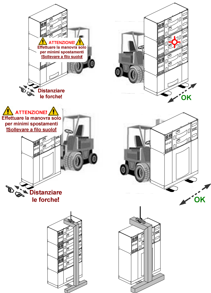
Figura 9-6: Movimentazioni ammesse
