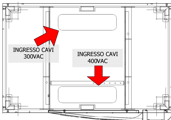
Figura 10-4: Passaggio cavi AC per sistemi \geq 275\text{kW} "ACbox-Trasformatore"
