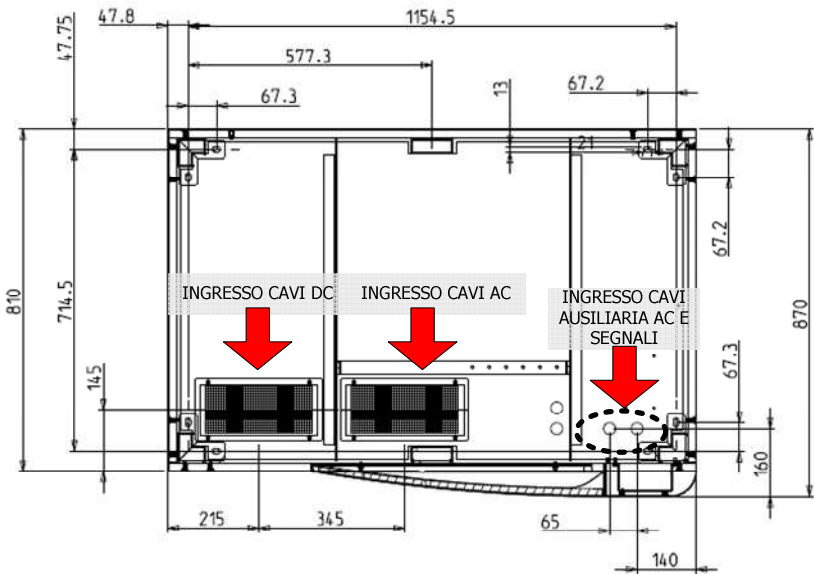
Figura 10-2: Fori passaggio cavi per sistemi con Trasformatore ≤220kW
