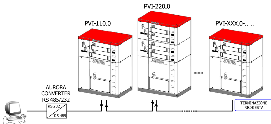
Figura 8-1: Modalità di passaggio del cavo seriale PVI-XXX.0
