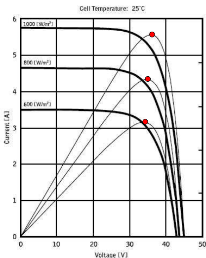
Figura 4-8: Esempio di curve I-V (Corrente-Tensione) e P-V (Potenza-Tensione) di un pannello solare
