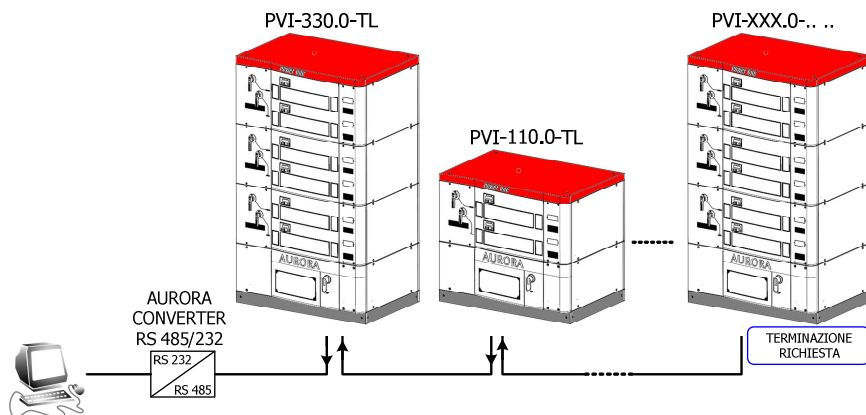
Figura 8-2: Modalità di passaggio del cavo seriale PVI-XXX.0-TL
