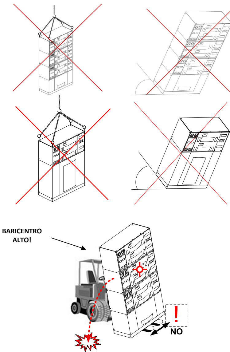
Figura 9-5: Movimentazioni non ammesse
