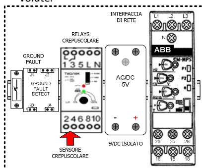
Figura 11-9: Relay Crepuscolare (versioni con Trasformatore di potenza \leq 220\text{Kw} )
