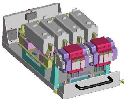
Figura 17-3: Cassetto DC
