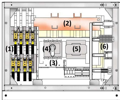
Figura 10-10: Composizione Zona ACBOX (versioni con Trasformatore \leq 220\text{kW} )
