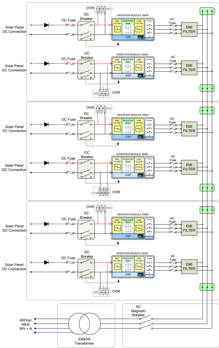
Figura 4-6: Schema elettrico di massima del PVI-XXX.0 con Trasformatore (versioni 275kW e 330kW)
