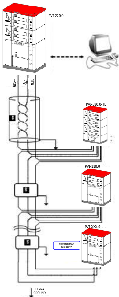
Figura 8-3: Tipologia di connessione dei PVI-XXX.0(-TL)
