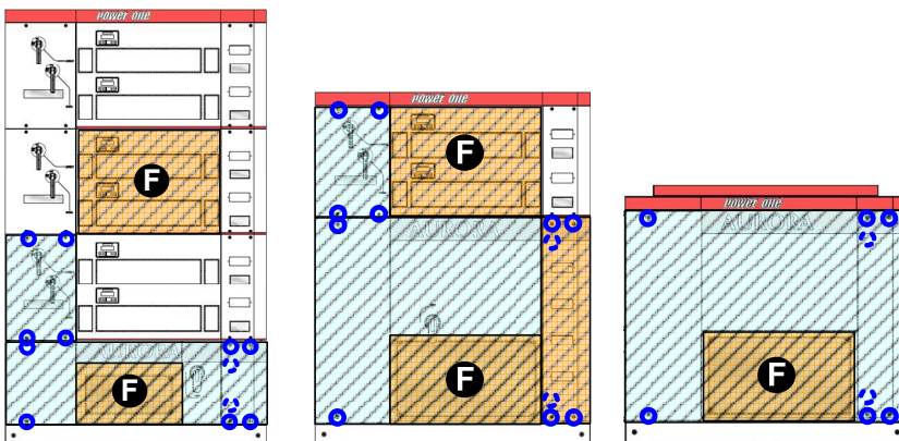
Figura 10-9: Pannelli da rimuovere
