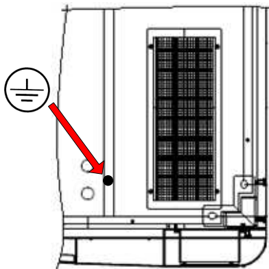
Figura 11-3: Collegamento del cavo di Terra di protezione (PE) per ACBOX senza Trasformatore
