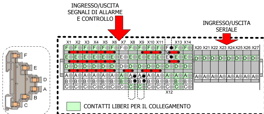
Figura 11-11: Morsettiera interna zona ACBOX
