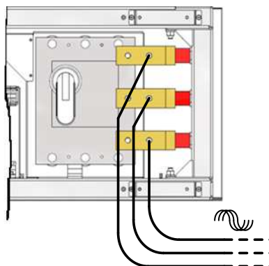
Figura 11-5: Collegamento cavi AC di potenza (versioni con potenza \geq 275\text{kW} o senza Trasformatore)
