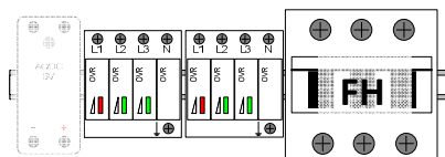
Figura 16-8: Dispositivi OVR AC per versioni senza trasformatore o \geq 275\text{kW}
