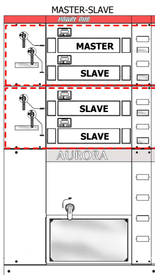
Figura 6-6: Composizione PVI-220.0 (1 Master-N.Slave)
