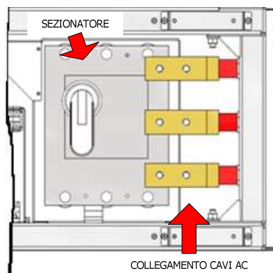
Figura 5-11: Ingresso Cavi AC (versioni con potenza \geq 275\text{kW} o senza Trasformatore)
