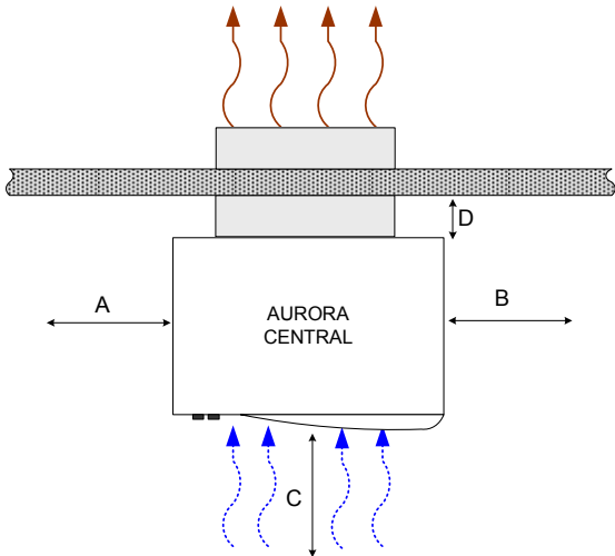
Figura 10-7: Distanze di rispetto
