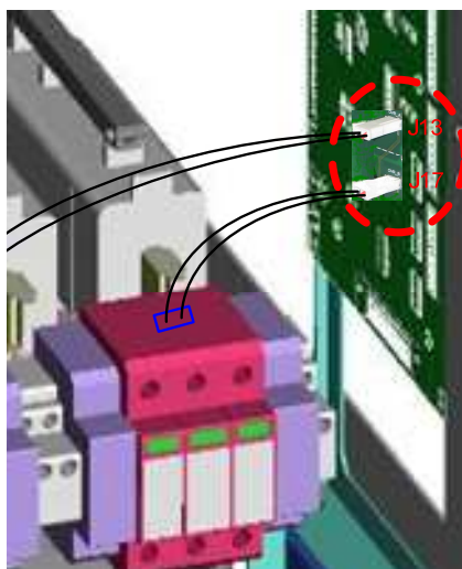
Figura 17-1: Collegamento del cassetto DC alla scheda
