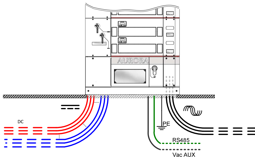
Figura 10-13: Uscita cavi sotto l'inverter (versioni senza Trasformatore)
