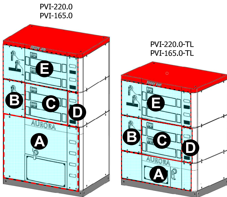
Figura 5-2: Vista generale del PVI-XXX.0(-TL) (versioni inferiori a 220kW 1 )
