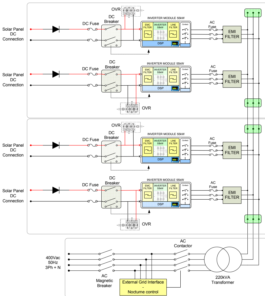
Figura 4-5: Schema elettrico di massima del PVI-XXX.0 con Trasformatore a bordo (≤220kW)
