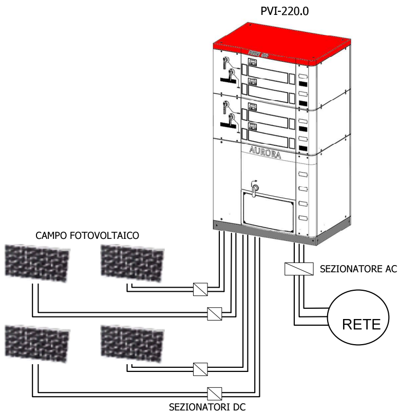
Figura 4-3: Esempio di collegamento alla rete AC dell'inverter con Trasformatore a bordo
