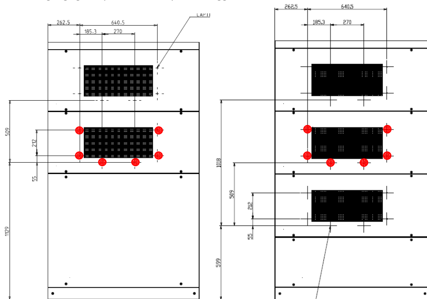
Figura 10-5: Griglie posteriori di areazione 1
