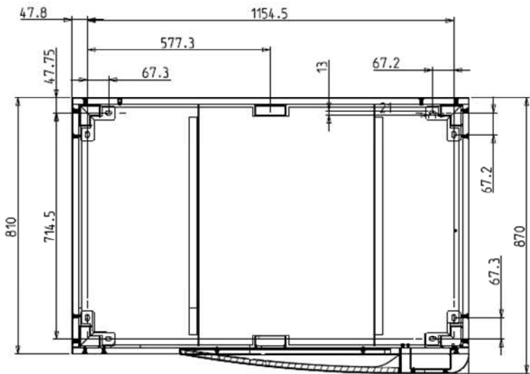
Figura 10-1: Footprint della base (uguale per tutti i sistemi)
