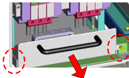
Figura 17-2: Viti di tenuta cassetto DC
