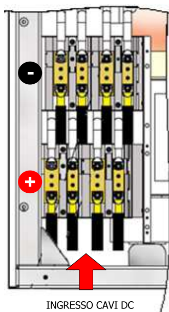
Figura 5-5: Ingresso Cavi DC (versioni con Trasformatore \leq 220\text{kW} )
