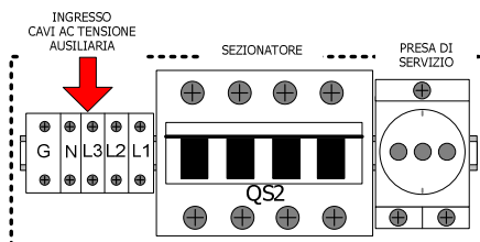
Figura 11-8: Morsetti di collegamento rete AC ausiliaria e relativo interruttore magnetotermico (versioni con Trasformatore di potenza \leq 220\text{kW} )
