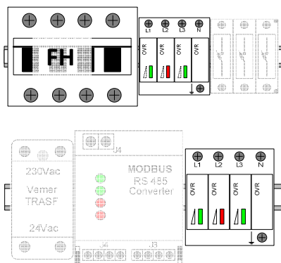
Figura 16-7: Dispositivi OVR AC per versioni con trasformatore \leq 220\text{kW}
