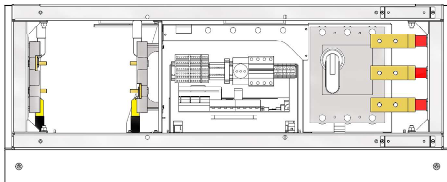
Figura 5-4: Vista generale ACBOX (A) (versioni con potenza \geq 275\text{kW} o senza Trasformatore)
