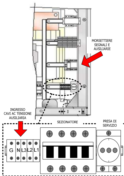
Figura 5-7: Ingresso Tensione Ausiliaria AC (versioni con Trasformatore \leq 220\text{kW} )
