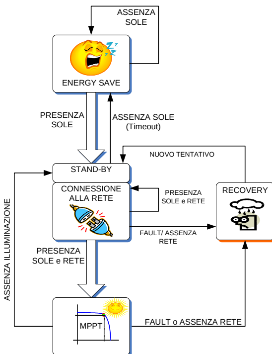
Figura 12-1: Diagramma di funzionamento dell'inverter
