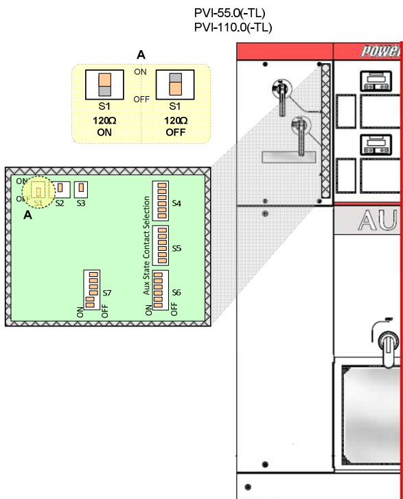
Figura 11-12: Posizione switch terminazione 120 ohm
