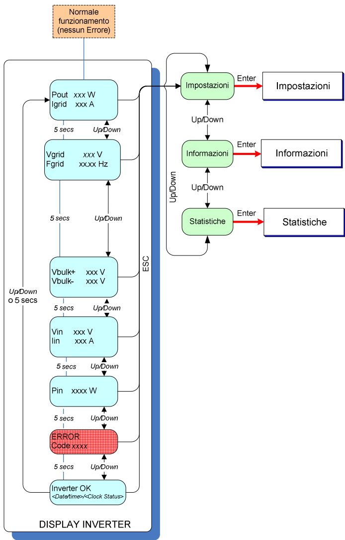
Figura 13-2: Diagramma funzionale del display (menù principale)
