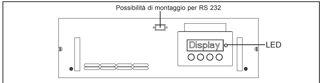
Fig. 5 Rack opzionale con display e LED
