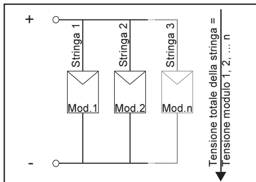
Fig. 2 Moduli solari in parallelo
