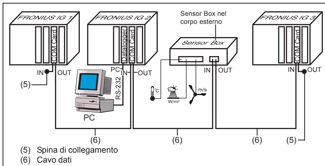
Fig. 6 Esempio di comunicazione dati tramite la LocalNet
