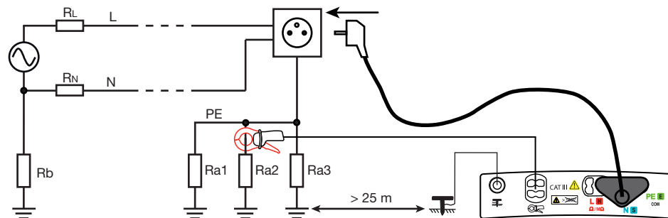
Caso di un impianto TT
